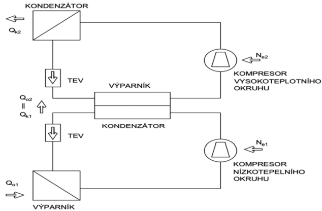
Obrázek 16 Jednoduché schéma kaskádního okruhu zapojení [1]
