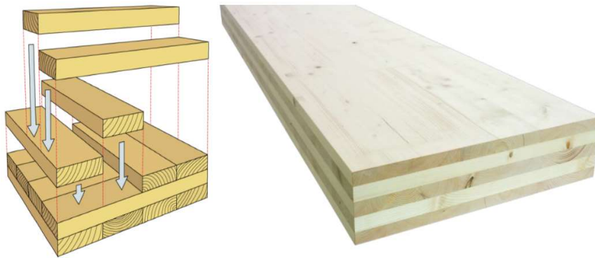
Obrázek 8 – Znárodnění kladení lamel a ukázka finálního produktu CLT panelu 49
