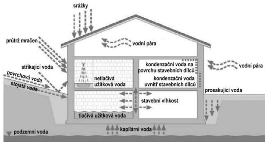
Obrázek 13 – Typická zatížení budov vlivem vlhkosti 116
