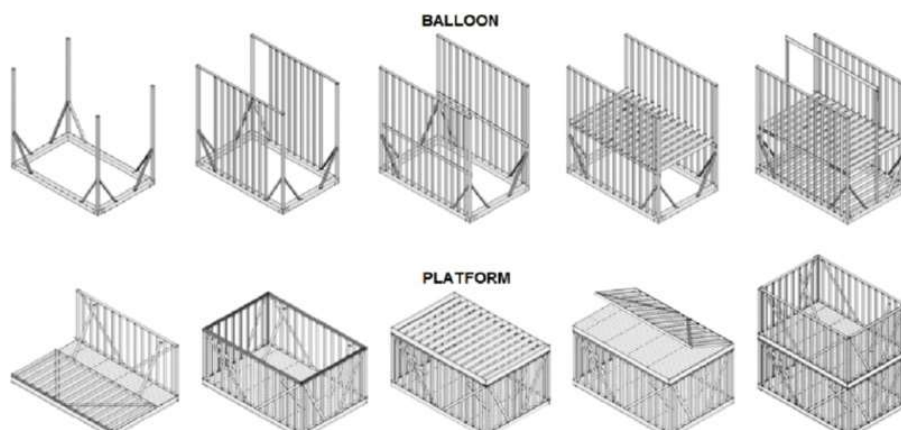
Obrázek 5 – Model výstavby Balloon-Frame a Platform-Frame 23
