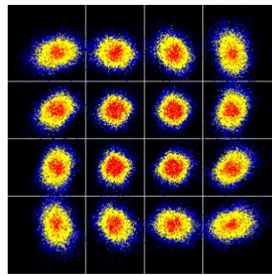
(d)MER=17.4 dB
