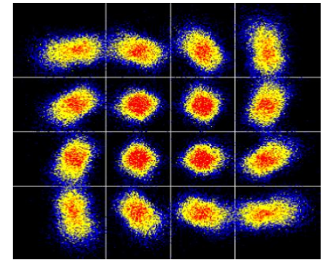
(d)MER=16.1 dB
