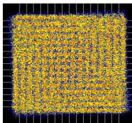
(d)MER=22.3 dB
