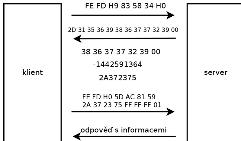
Obrázek 3.5: Příklad komunikace
