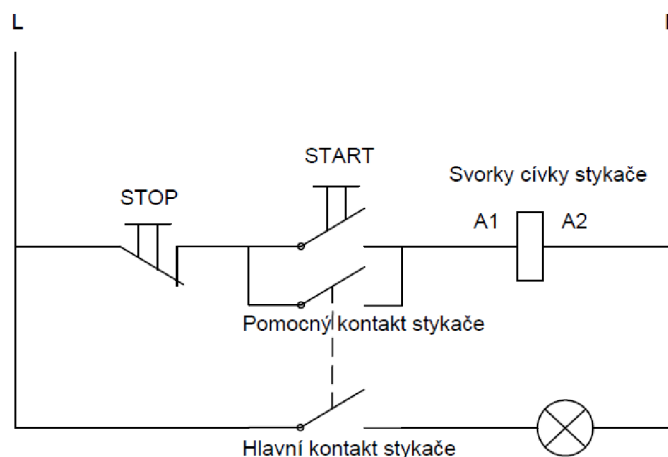
Obr. 4-1 Schéma typického zapojení stykače s dvoutlačítkem
