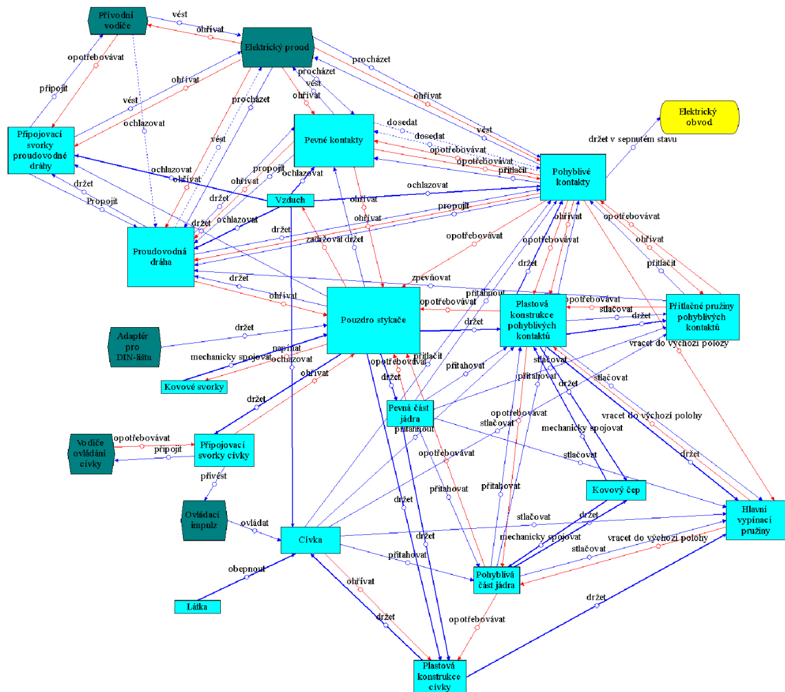
Obr. 5-1 Model funkcí stykače v sepnutém stavu
