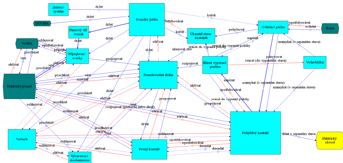
Obr. 5-6 Model funkcí jističe v sepnutém stavu
