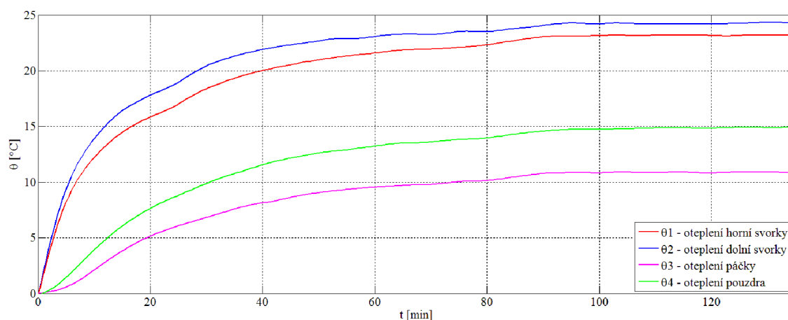
Graf 8-9 Průběh oteplení jističe 1 při 3. měření
