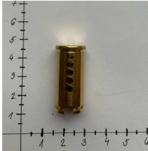
Obr. č. 10 cylindr cylindrické vložky zdroj: vlastní zpracování
