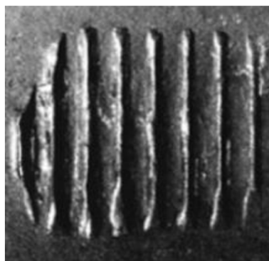
Obr. č. 32 - statická stopa (vtisk kleští)
