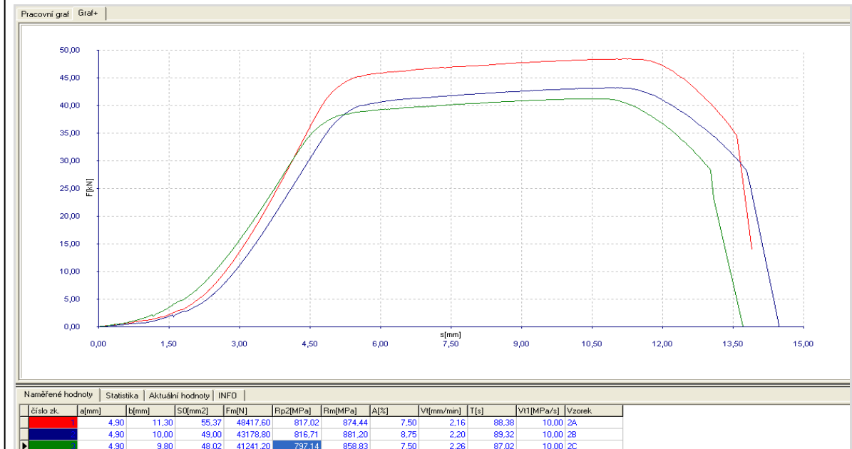
Obr. 36 Tahový diagram nátavu 8.
