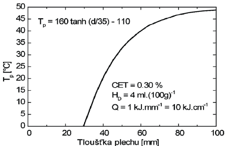
„Obr. 8 Závislost tloušťky plechu ( d ) na výši teploty předehřevu ( T_p ) pro CET 0,30% "[2]
