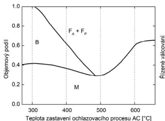
„Obr. 5 Závislost objemového podílu mikrostrukturních fází na teplotě zastavení ochlazovacího procesu/ (AC) "[2]
