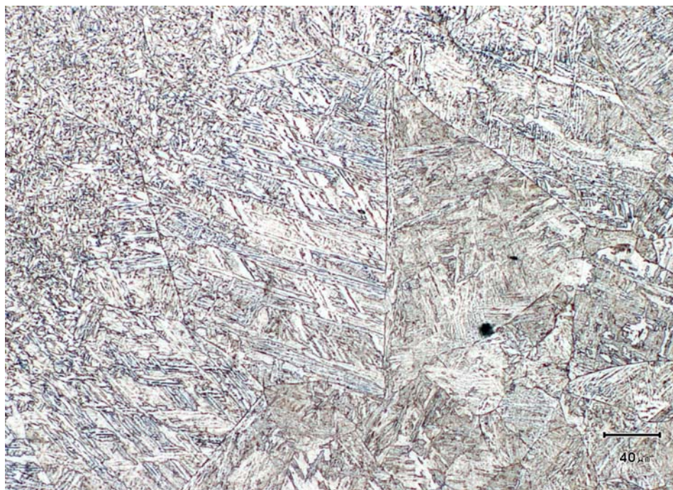
Obr. 45 Někteřá zřna v přehřátém pásmu TOO v blízkosti hranice zřavení mají v průměřu až 0,3 mm. Leptáno Nitalem 1%.
