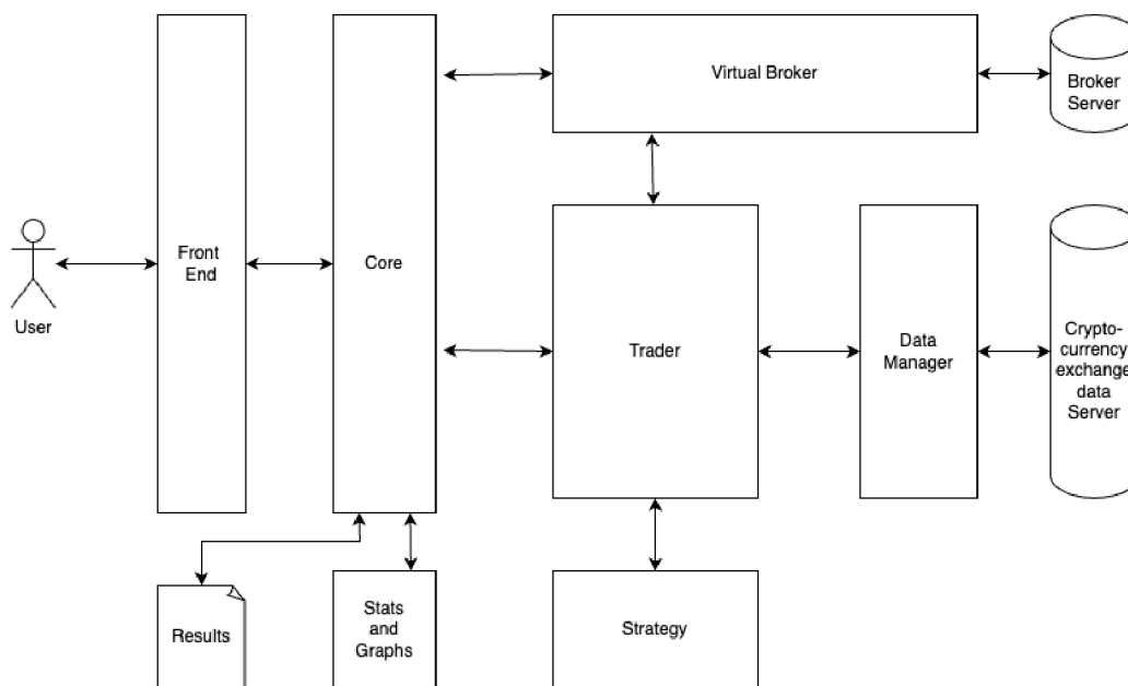
Obrázek 3.1: Diagram architektury AOS.
