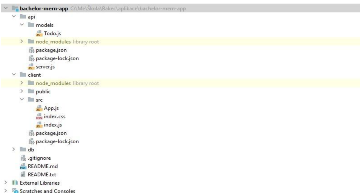
Obr. 1: Struktura MERN aplikace (vlastní zdroj)
