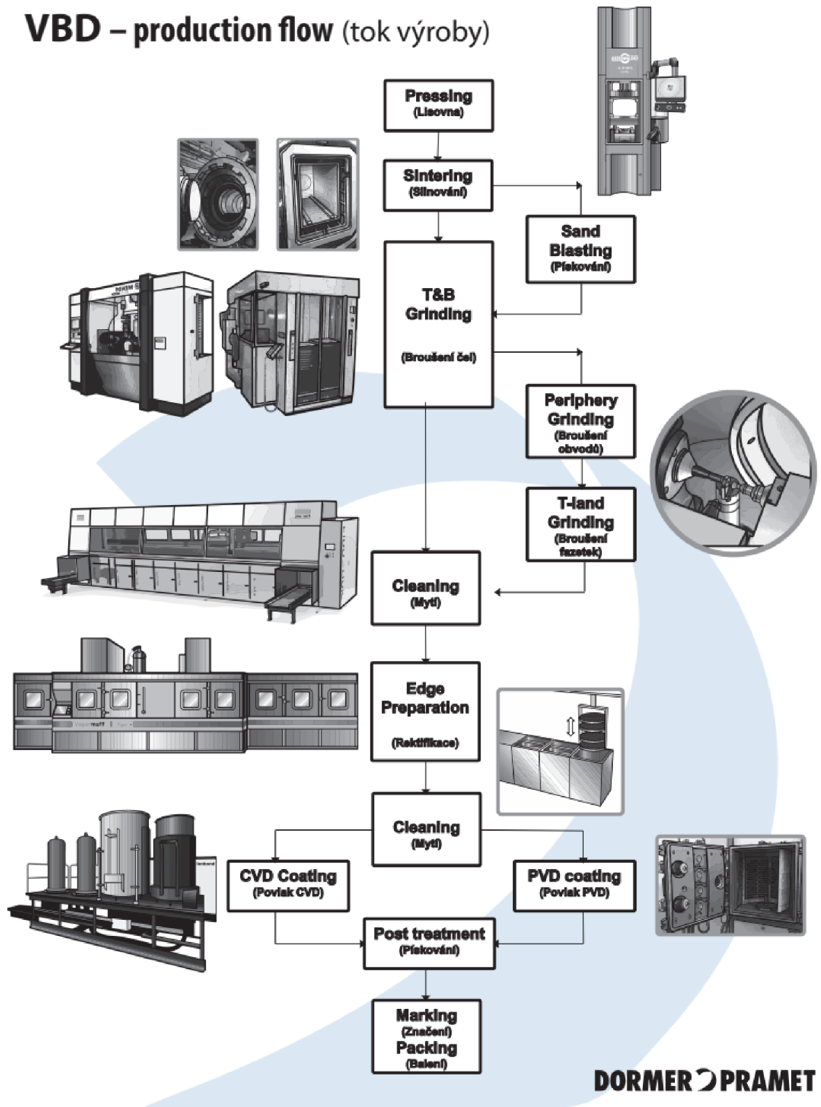
obr. 4 Tok výroby – pracoviště lisovny, Dormer Pramet [3]
