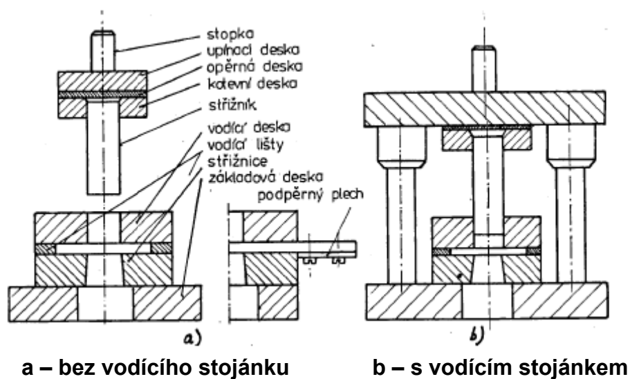
Obr 4.9 Střížný nástroj
