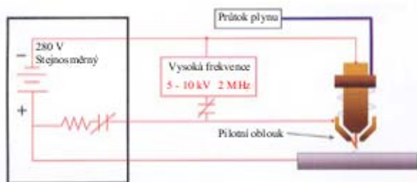
Obr. 6.4 Pilotní oblouk
