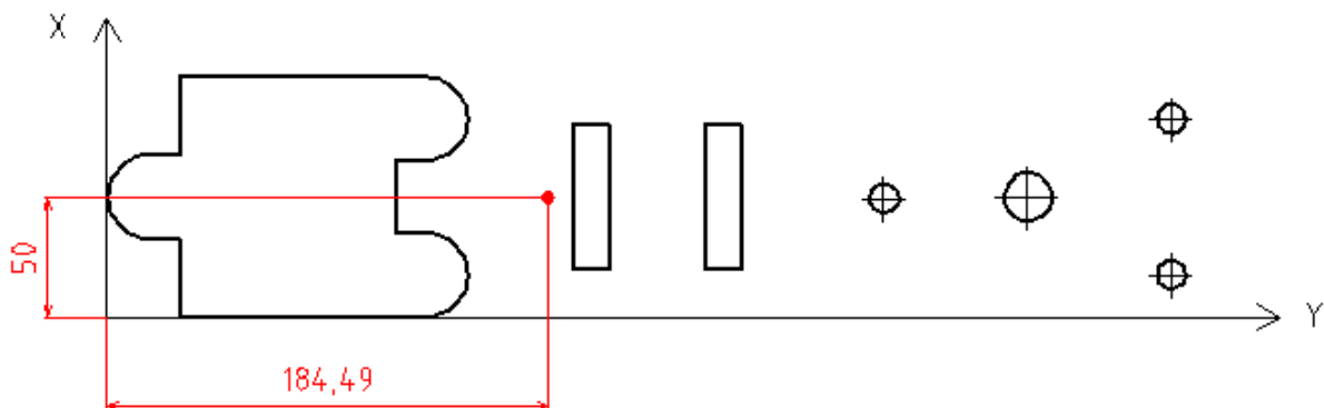
Obr. 4.7 Těžiště střížných sil
