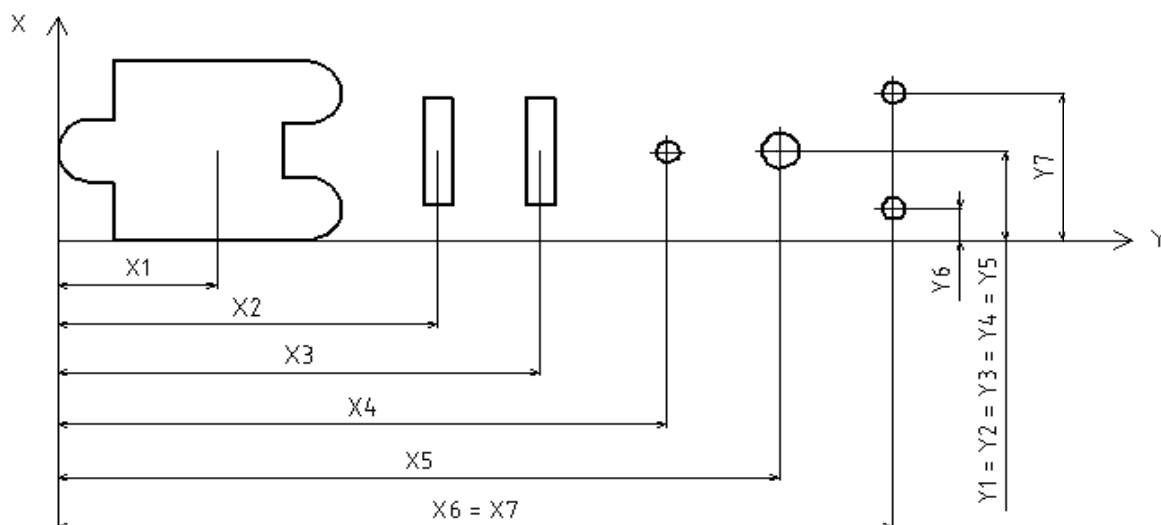
Obr. 4.2 Souřadnice os
