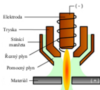
Obr. 6.7 Plazmový řez dvěma plyny
