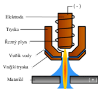
Obr. 6.9 Řezání s injekcí vody
