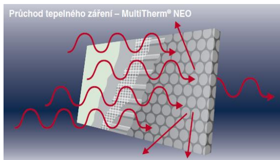
Obr. 7 – Průchod tepelného záření šedým polystyrenem [18]
