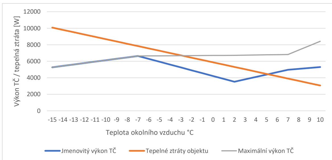
Obr. 29 – Průběh TZ objektu se zateplením var. 3 a char. výkonů TČ AWB-M-E-AC 221.C8
