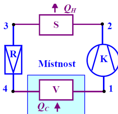
Obr. 22 – Schéma zapojení TČ a funkce jednotlivých součástí v režimu chlazení [53]
