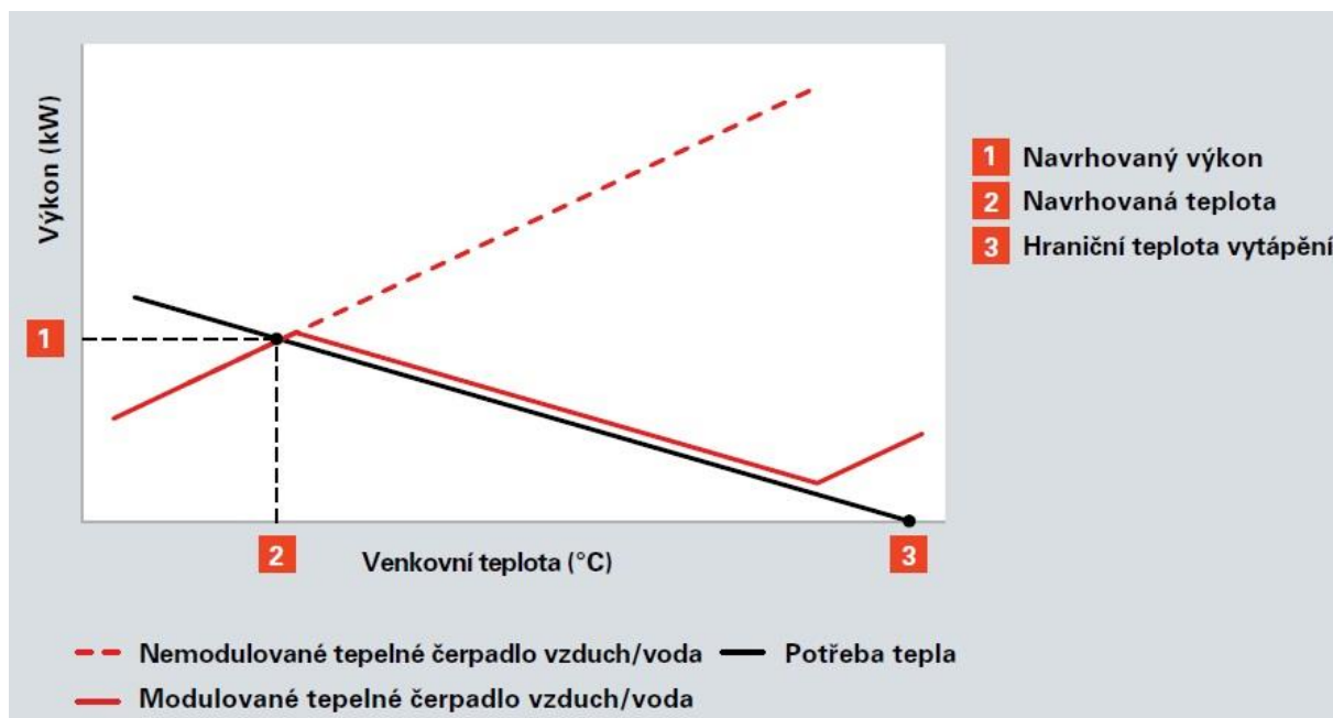
Obr. 24 – Regulace tepelného výkonu TČ vzduch/voda [47]
