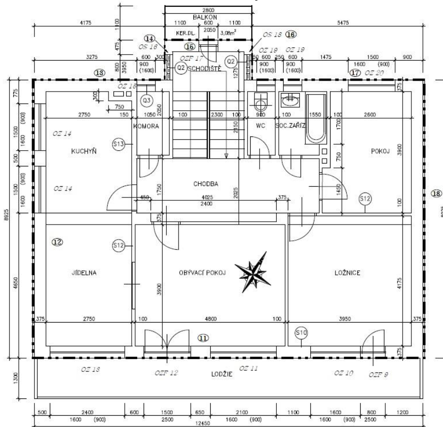
Obr. 28 – Půdorys 2NP
