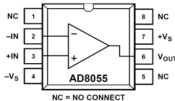
Obr. 9: Rozmístění vývodů obvodu AD8055
