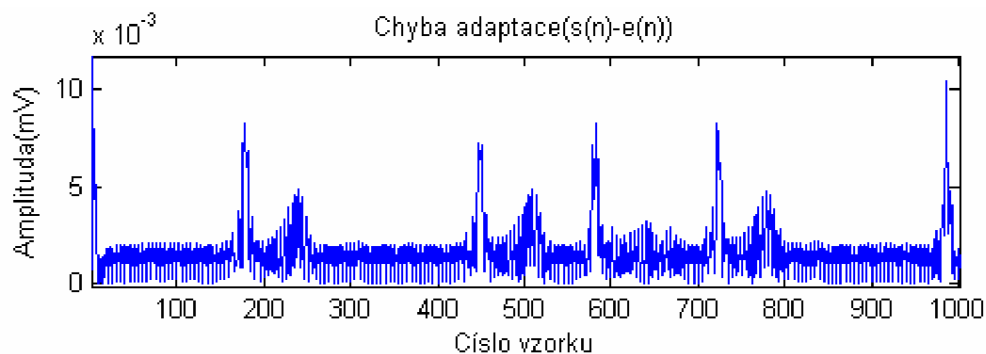
Obrázek 47: Chyba adaptace uvedená v absolutních hodnotách pro systém uvedený v kapitole 4.4
