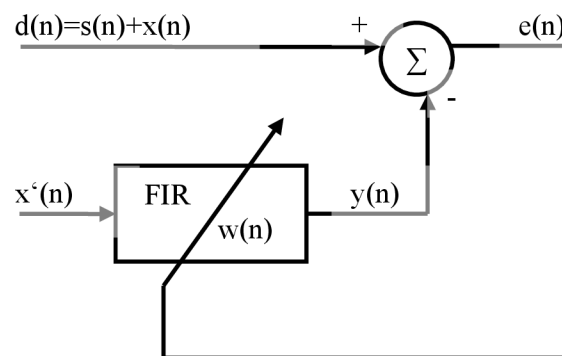
Obrázek 16: Vstupní signál d(n) je složený z užitečného signálu s(n) (signál EKG) a uměle vytvořeným šumem x(n) je zaručen. Referenční signál x'(n) je šum.
