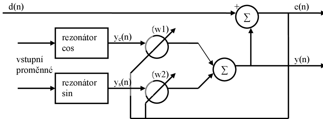
Obrázek 19: Blokové schéma úzkopásmové adaptivní zadrž s využitím číslicového rezonátoru
