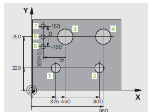
Obr. 24: Příklad absolutního a relativního vztažného bodu (16, s. 102)
