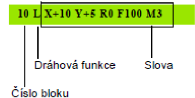
Obr. 25: Prvky bloku (16, s. 103)
