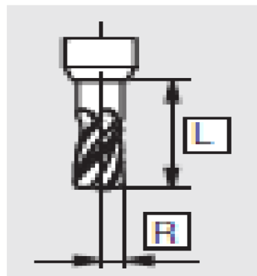
Obr. 31: Délka a rádius nástroje (16, s. 176)
