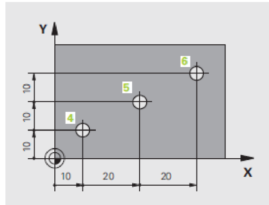
Obr. 23: Díry s inkrementálními souřadnicemi (16, s. 101)
