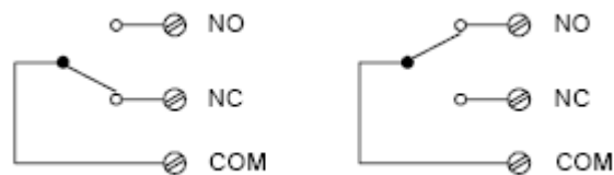
Obr. 12: Funkce přepínačů na reléové kartě
