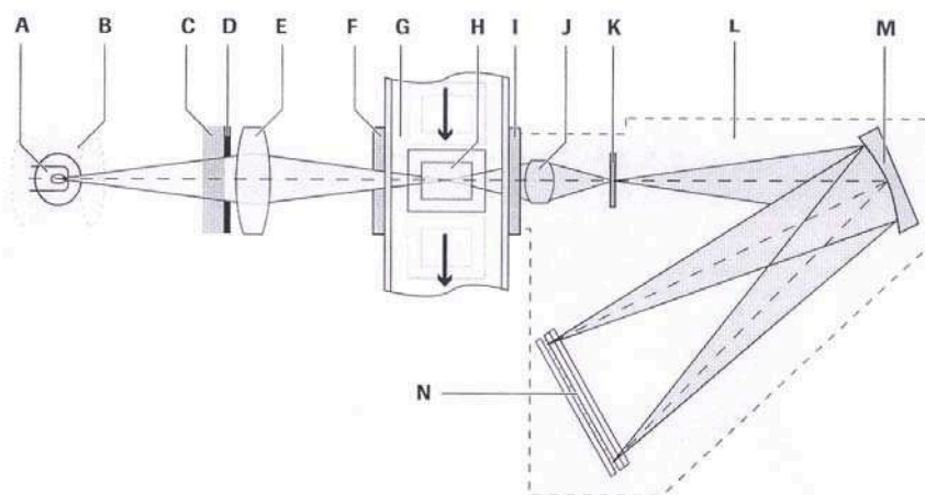
Obr. č. 10 Optická dráha fotometru modulu c501 systému Cobas 6000, Roche [39]
