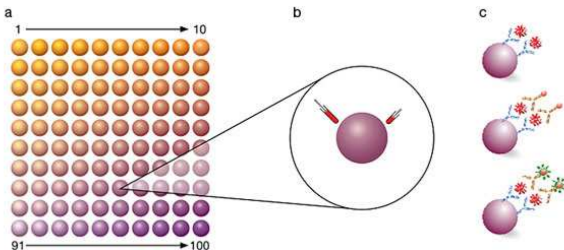
Obr. č. 4 Multiplexová imunoanalýza: uvnitř mikročastice jsou dvě různé fluorescenční barviva (červené a infračervené). K výrobě 100 barevně kódovaných sad mikročastic se používá deset různých koncentrací červeného a infračerveného barviva. Každá mikročastice je schopna specificky vázat určitý analyt (a). Ten pak reaguje s biotinylovanou protilátkou (b), na kterou se naváže konjugát streptavidin – phycoerytrin (c) [32]
