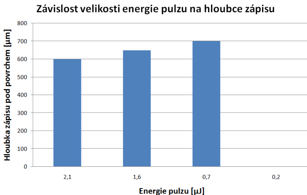
Obr. 7.6: Závislost velikosti energie pulsu na hloubce zápisu pod povrchem
