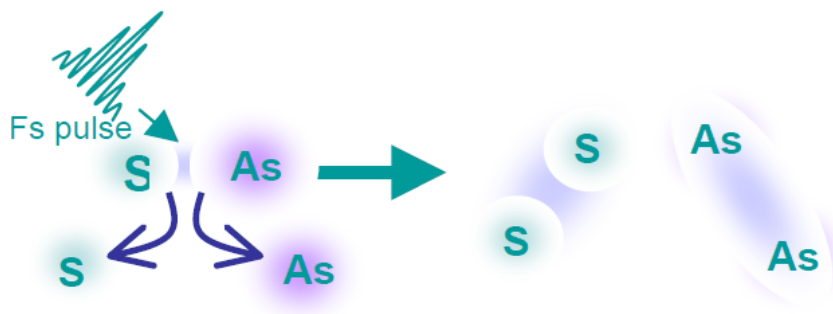
Obr. 5.2: Restrukturalizace vazby v \text{As}_2\text{S}_3 pomocí femtosekundového laseru [13]
