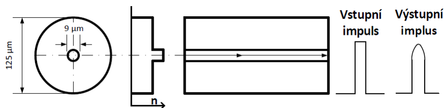
Obr. 2.1: Jednovidové optické vlákno
