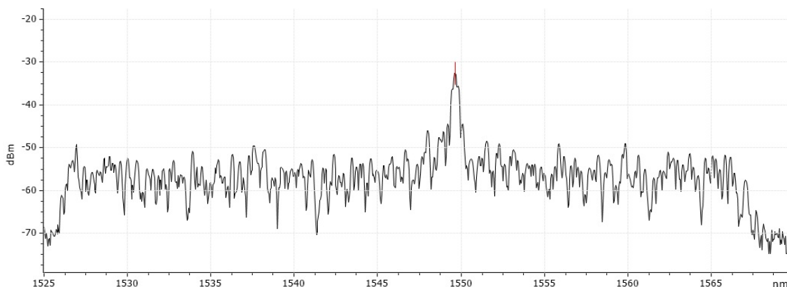
Obr. 7.15: Odražené spektrum Braggovy mřížky
