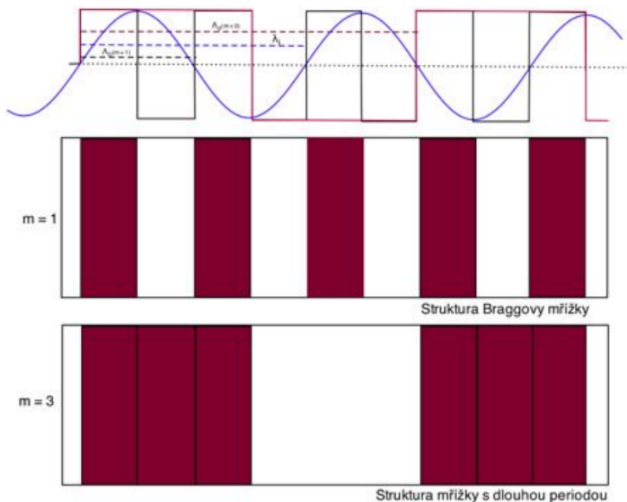
Obr. 3.7: Porovnání Braggovy mřížky a mřížky s dlouhou periodou [7]
