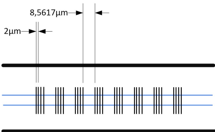
Obr. 7.13: Metoda dvou period
