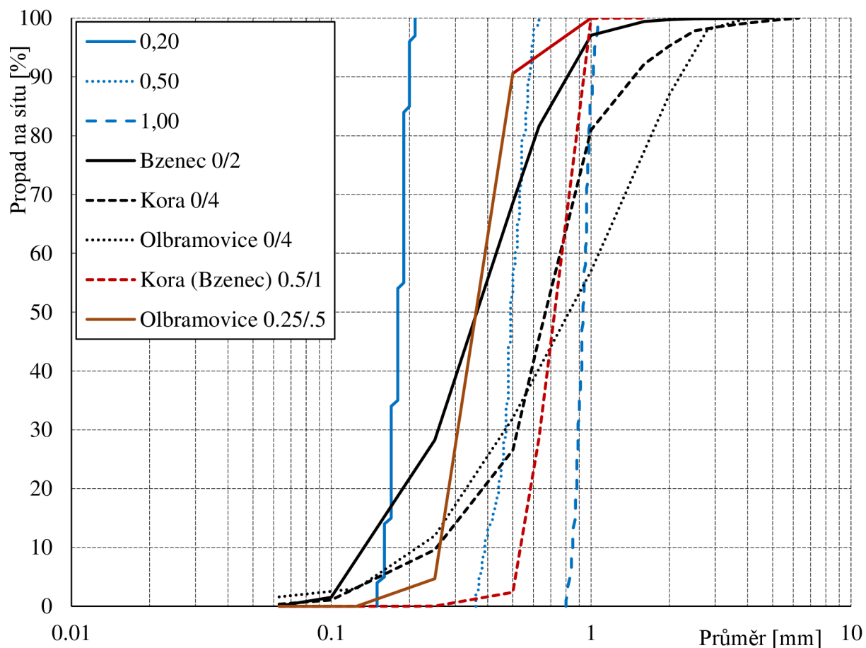
Obr. 3.2 Křivky zrnitosti
