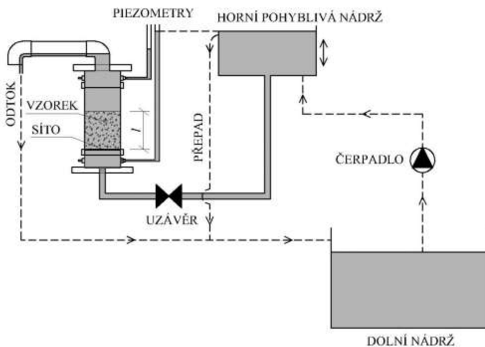
Obr. 3.4 Schéma měřícího zařízení
