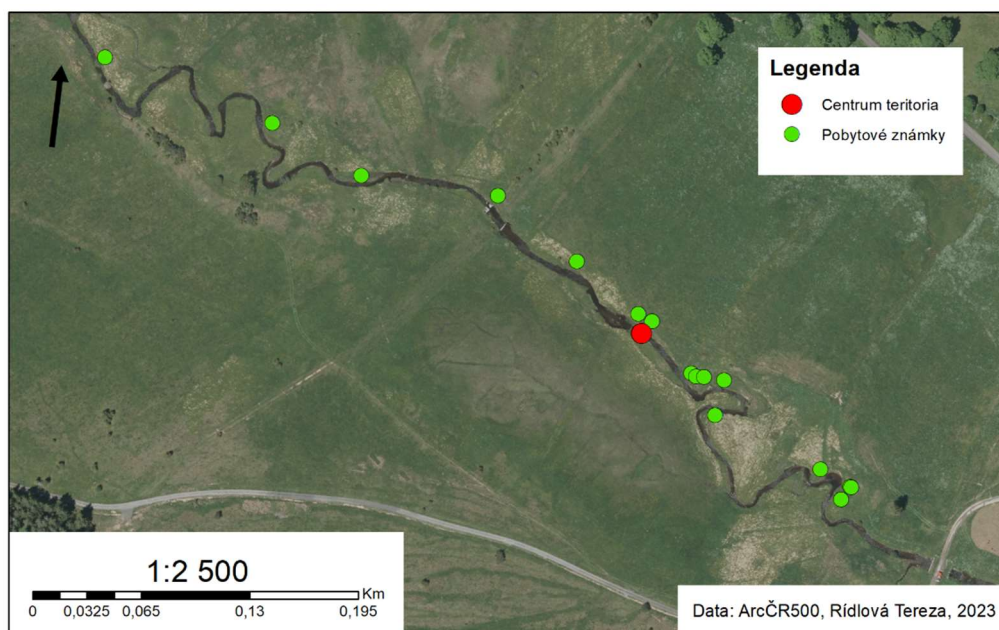
Obr. 7: Pobytové známky bobra a centrum teritoria na lokalitě Haďák
