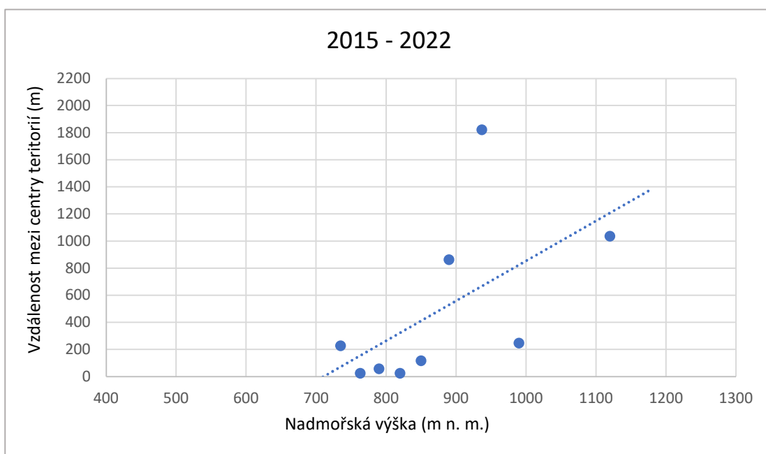
Graf 3: Posun center teritorií v letech 2019 – 2020 v různých nadmořských výškách
