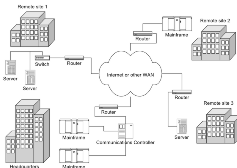
Obrázek 3: Architektura distribuované databáze [8]
