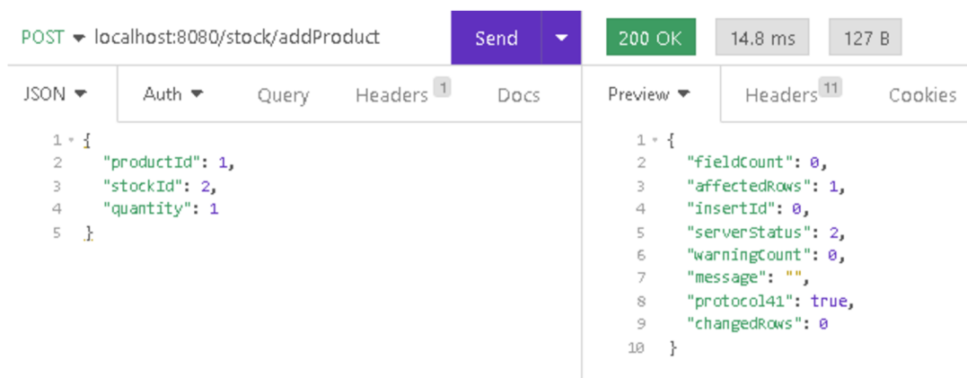
Obrázek 9: Požadavek v programu Insomnia rest client [autor]
