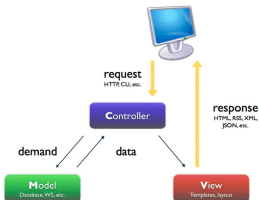
Obrázek 8: MVC architektura [41]
