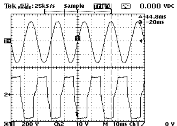
Graf č.10 I=10\text{A} , \text{Ch2}=\text{OZ3in} , R_6=0
