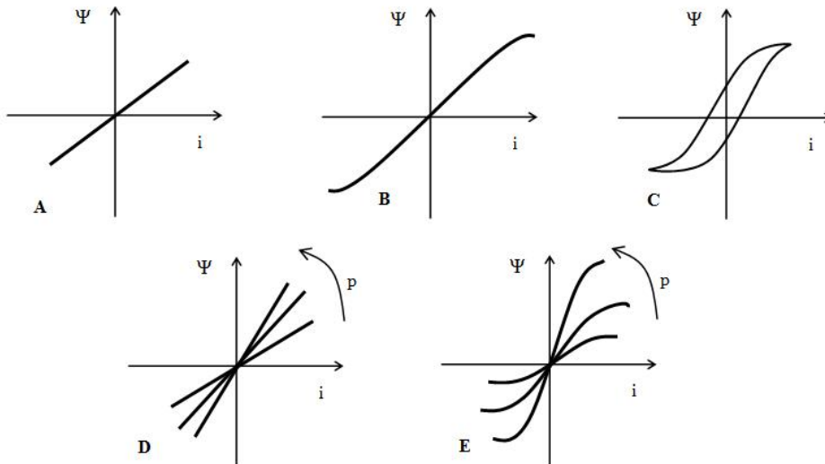
Obr.2.5.1-1 Magnetické obvody – A) lineární, B) Nelineární, C) Nelineární s hysterézí, D) Lineární parametrický, E) Nelineární parametrický
