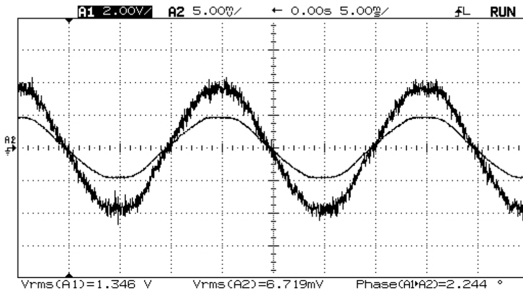
Graf č.27 A_2=I_1 ; A_1=U_{Rb} , I_1=40A , U=1,346V
