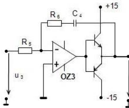
Obr.3.4-3 PI regulátor s emitorovým sledovačem
