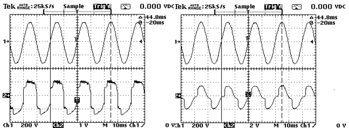
Graf č.15 I=10A , Ch2=OZ3out , R_6=6,7k
