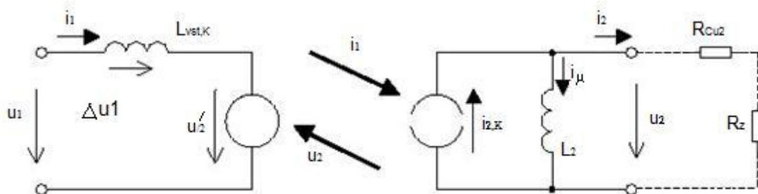
Obr.2.6.2-1 Obvodový model transformátoru proudu
