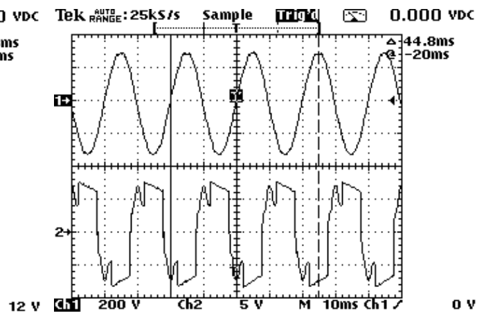
Graf č.4 I=10A , OZ3in , R_6=10k
