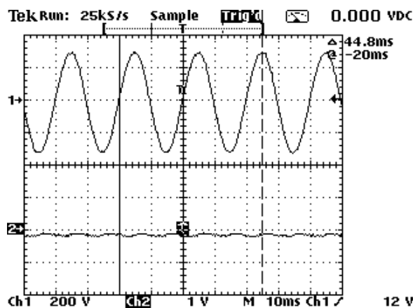
Graf č.1 I=10A , Ch2=OZ1out ,
