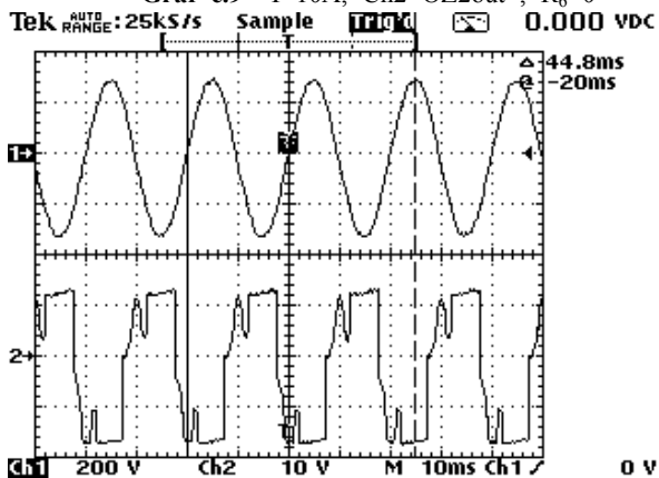
Graf č.9 I=10\text{A} , \text{Ch2}=\text{OZ2out} , R_6=0
