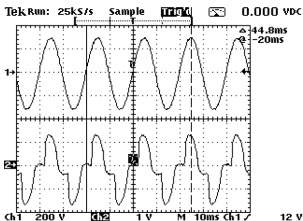
Graf č.3 I=10A , Ch2=U_{Rb} , R_6=0
