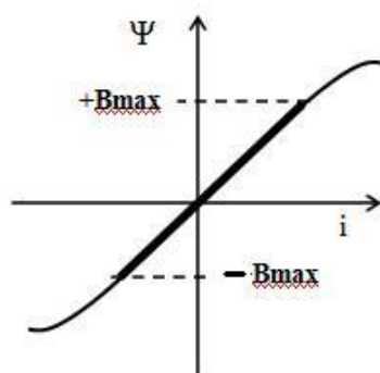
Obr.2.5.2-1 Magnetický obvod lineární
