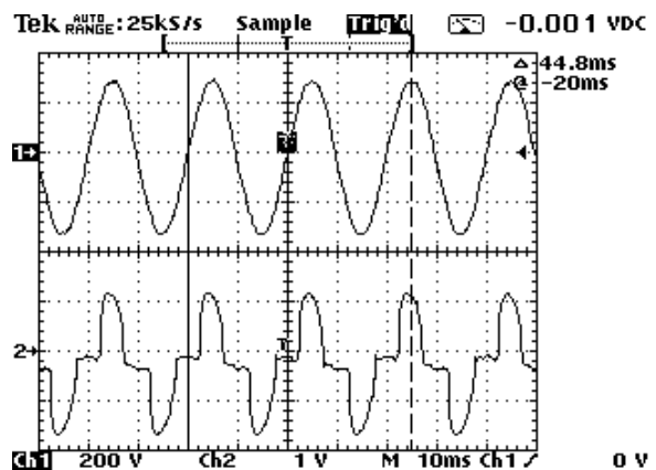
Graf č.12 I=10\text{A} , \text{Ch2}=\text{U}_{R_6} , R_6=40\text{k} , C=0
