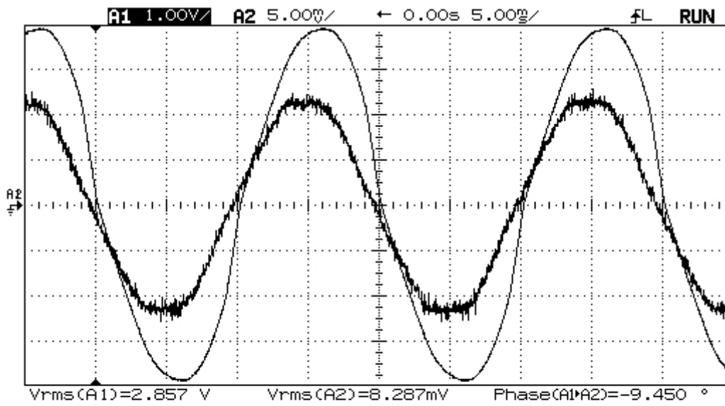
Graf č.23 A2 = I_1 ; A1 = U_{OZ3out} , I_1 = 50 \text{ A} , U = 2,857 \text{ V}
