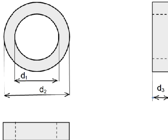
Obr.3.2.-1 Rozměry feritového jádra T3813, CF138
