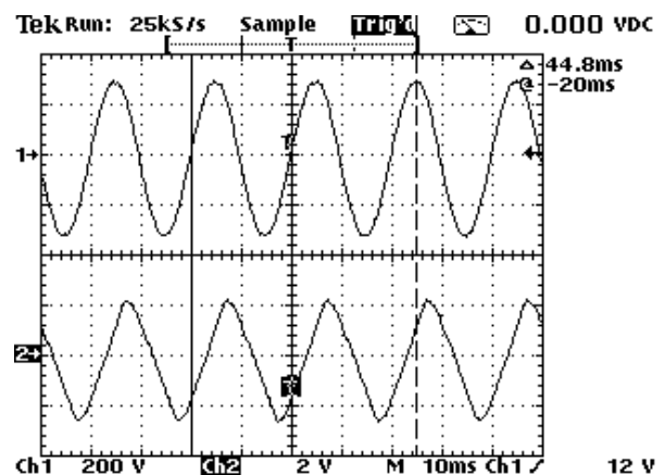
Graf č.2 I=10A , Ch2=OZ2out , R_6=0
