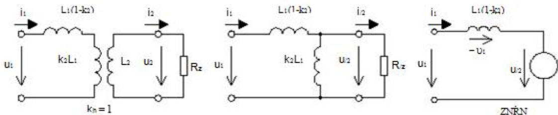
Obr.2.7.2-1 TR po T separaci. Náhradní zapojení T - článku
