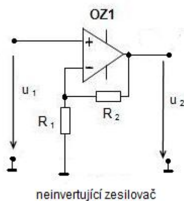
Obr.3.4-1 Neinvertující OZ
