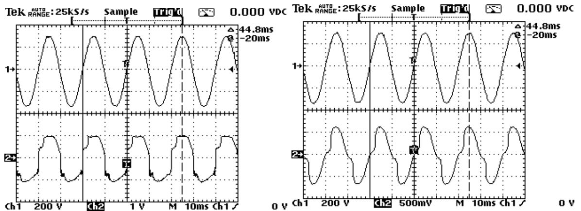
Graf č.13 I=4A , Ch2=OZ3out , R_6=6,7k
