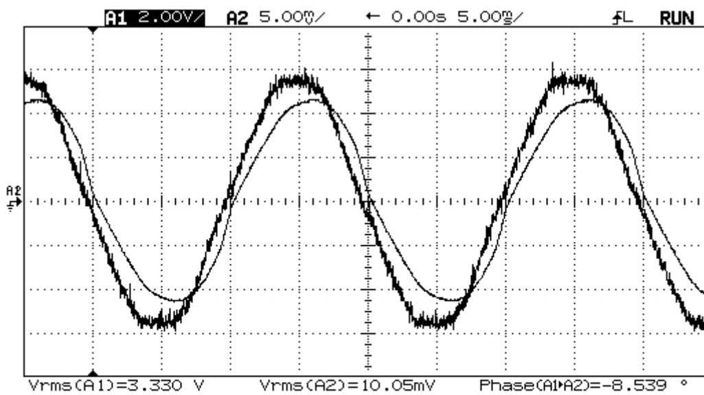
Graf č.24 A2 = I_1 ; A1 = U_{OZ3out} , I_1 = 60 \text{ A} , U = 3,330 \text{ V}
