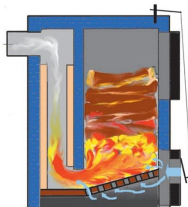
Obr.2.4: Odhořivací kotel[36]
