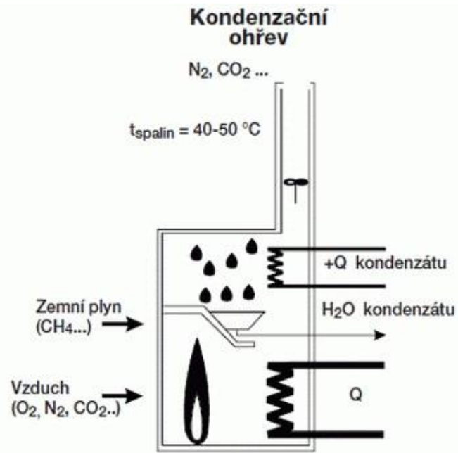
Obr.2.2: Kondenzační kotel[35]
