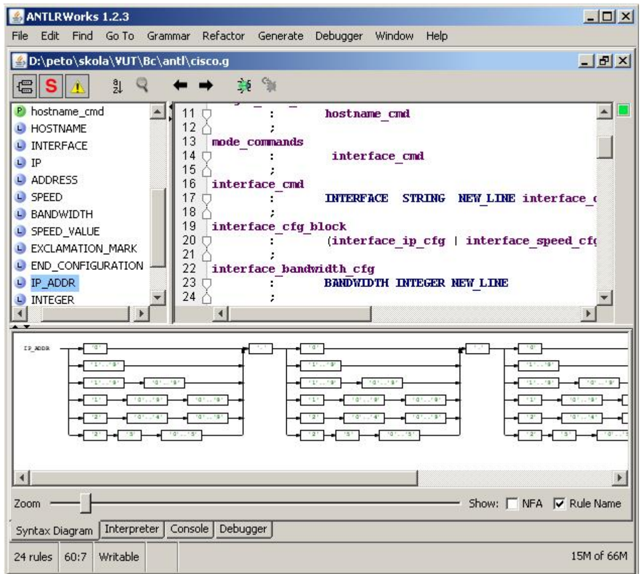
Obrázek 5.1: ANTLRWorks 1.2.3.
