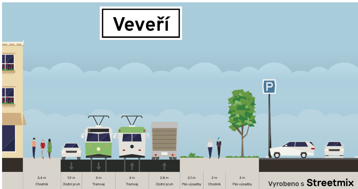
Obrázek 23: Schéma šířkového uspořádání ulice Veveří [26]
