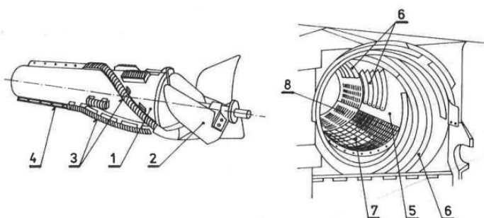
Obrázek 2.6: Schéma uspořádání axiálních mlátících a separačních bubnů (Břečka et al., 2001)
