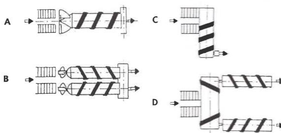
Obrázek 2.5: Schéma uspořádání axiálních mlátících a separačních bubnů (Břečka et al., 2001)
