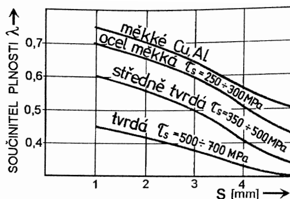
Obr. 33 Nomogram pro určení součinitele plnosti [3]
