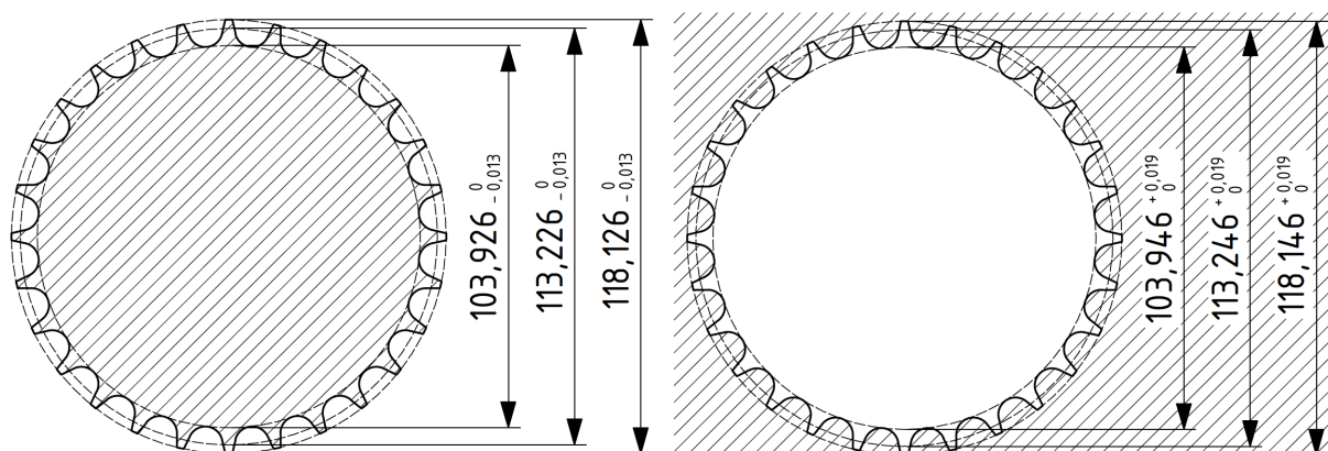
Obr. 35 Znáornění funkčních rozměrů nástroje pro vystřihování, vlevo - střížník, vpravo - střížnice
