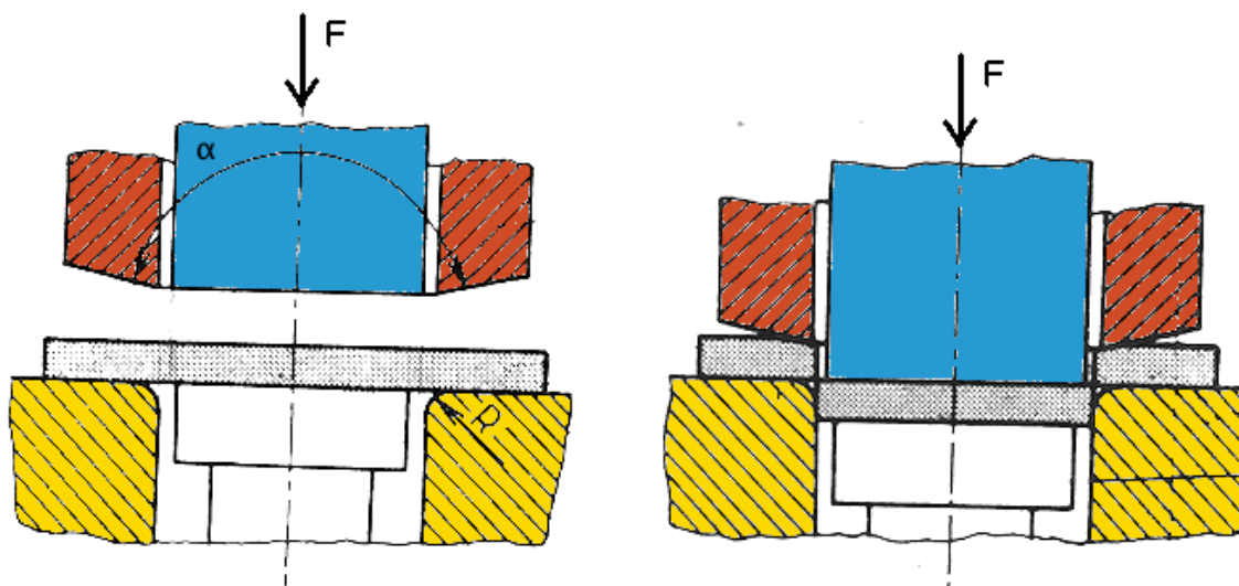
Obr. 12 Stříhání se zkoseným přidržovačem [7]
