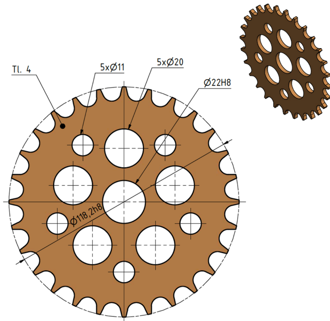
Obr. 2 Ozubené kolo
