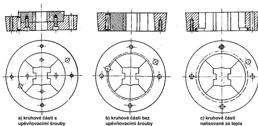
Obr. 22 Skládané střížnice [5]
