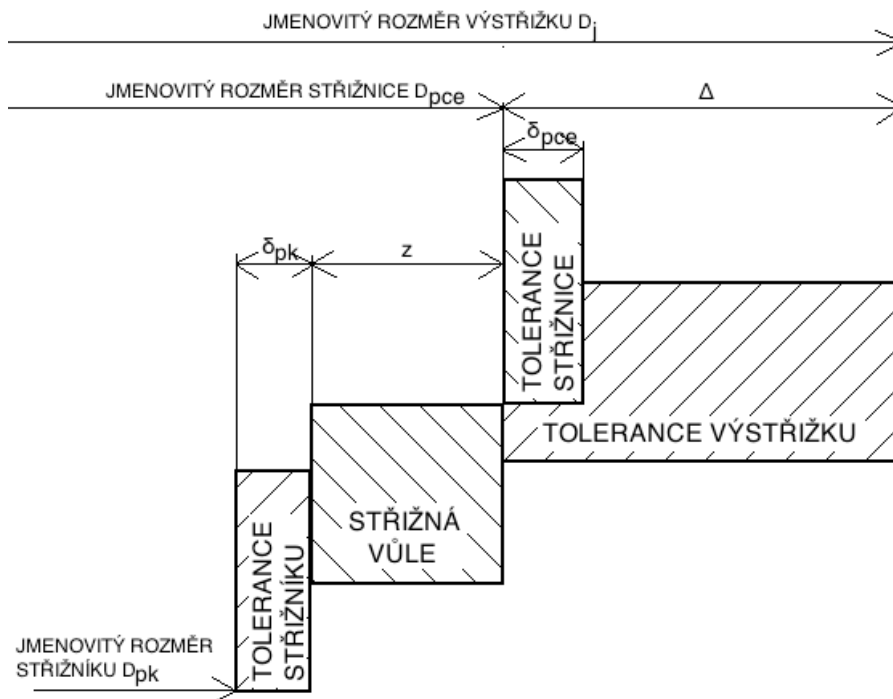
Obr. 34 Určení rozměrů střížníku a střížnice při vystříhování
