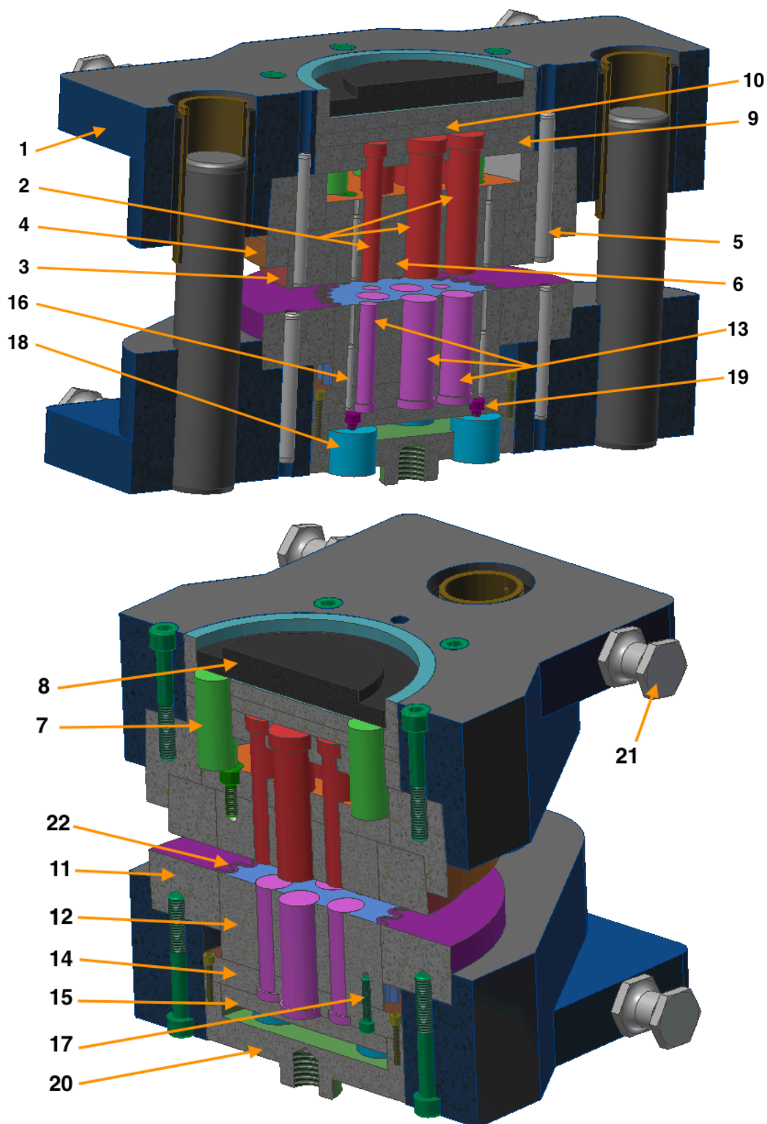
Obr. 38 Princip nástroje
