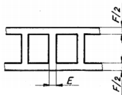
Obr. 27 Znárodnění můstku a postranního odpadu [3]
