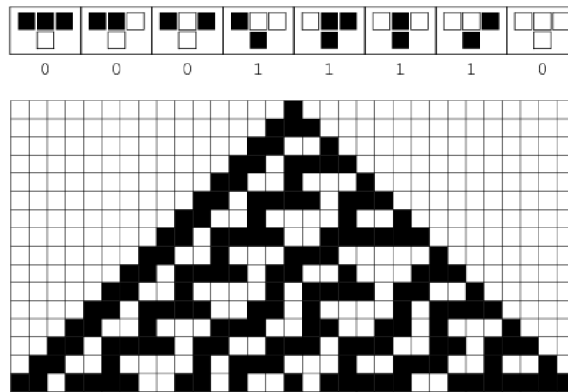
Obrázek 2.2: Graficky znázornené pravidlo 30 a začiatok vývoja celulárneho automatu
