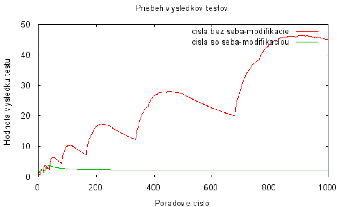
Obrázek 5.6: Postupne zaznamenané výsledky testu
