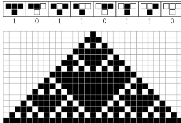
Obrázek 5.4: Graficky znázornené pravidlo 182 a začiatok vývoja celulárneho automatu
