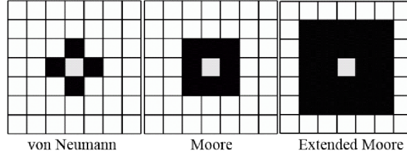
Obrázek 2.3: Rôzne druhy okolí dvoj-dimenzionálnych celulórnnych automatov
