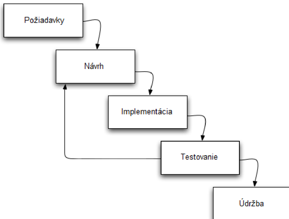
Obrázek 4.1: Vodopádový model
