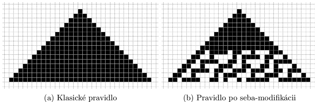
Obrázek 3.1: Znázornenie seba-modifikácie
