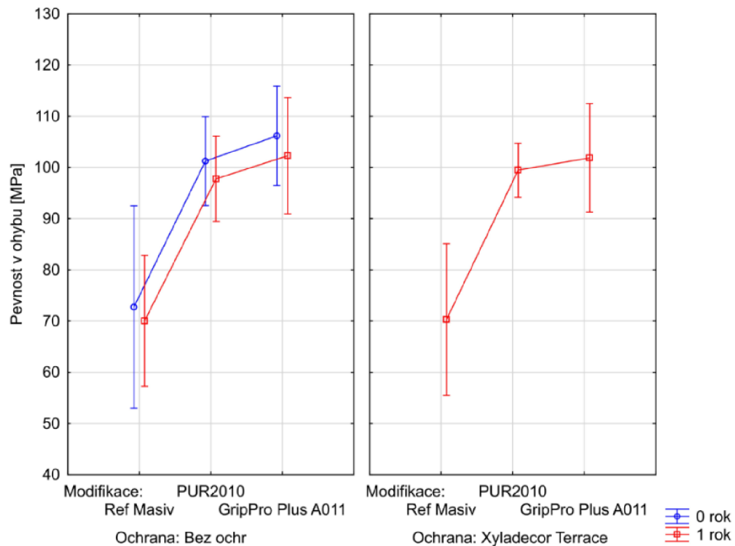
Graf 3: Síla závislosti pevnosti v ohybu lepeného lamelového dřeva dubu při různých úpravách (Zdroj: Autor práce)
