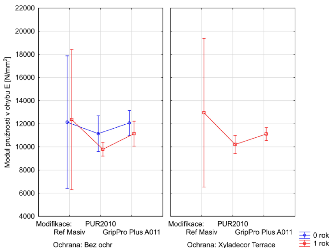
Graf 4: Globální E modul pružnosti v ohybu lepeného lamelového dřeva dubu při různých úpravách (Zdroj: Autor práce)
