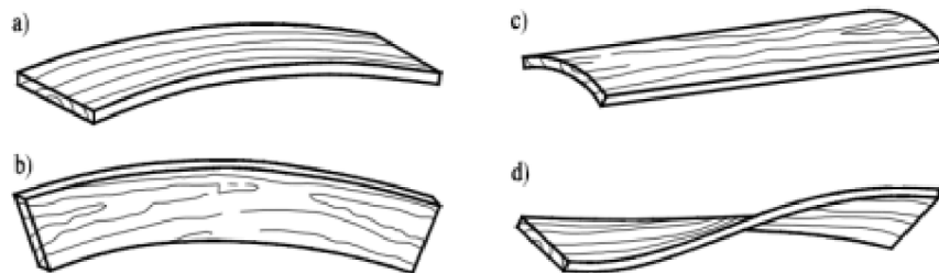
Obrázek 4: : Podélné borcení dřeva a) podélné plošné borcení, b) podélné boční borcení, c) příčné borcení, d) šroubovitě borcení (Zdroj: Svoboda 2013)
