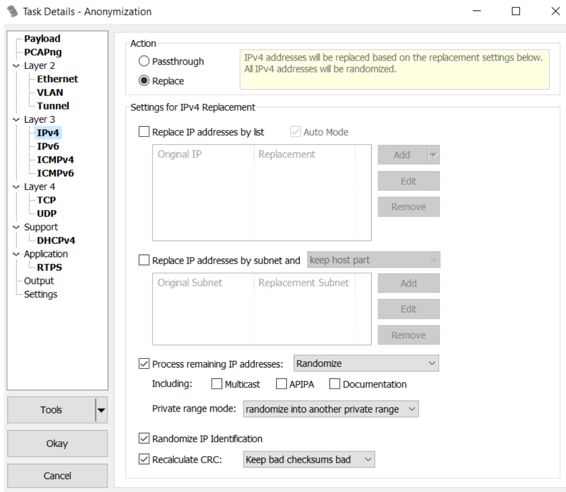
Obr. 4.2: Nastavenie anonymizácie v programe TraceWrangler
