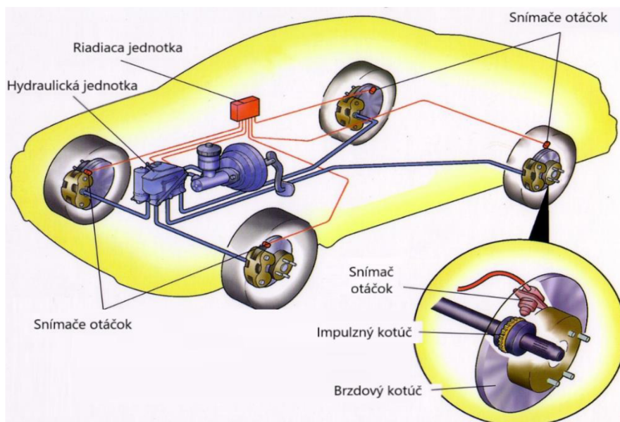
Obr. 3 Protiblokovací systém ABS v automobile [6]
