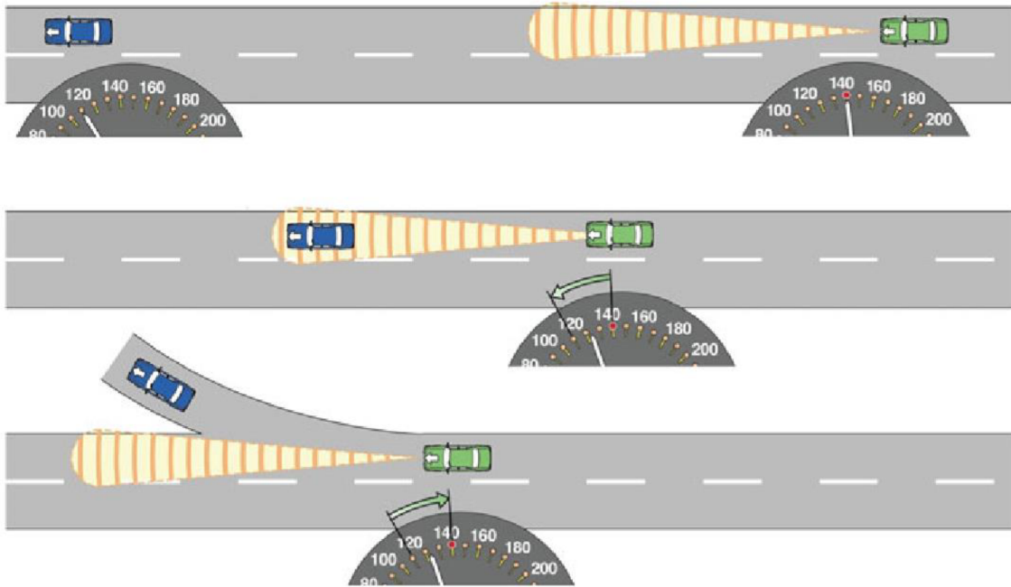
Obr. 8 Funkcia adaptívneho tempomatu [3]
