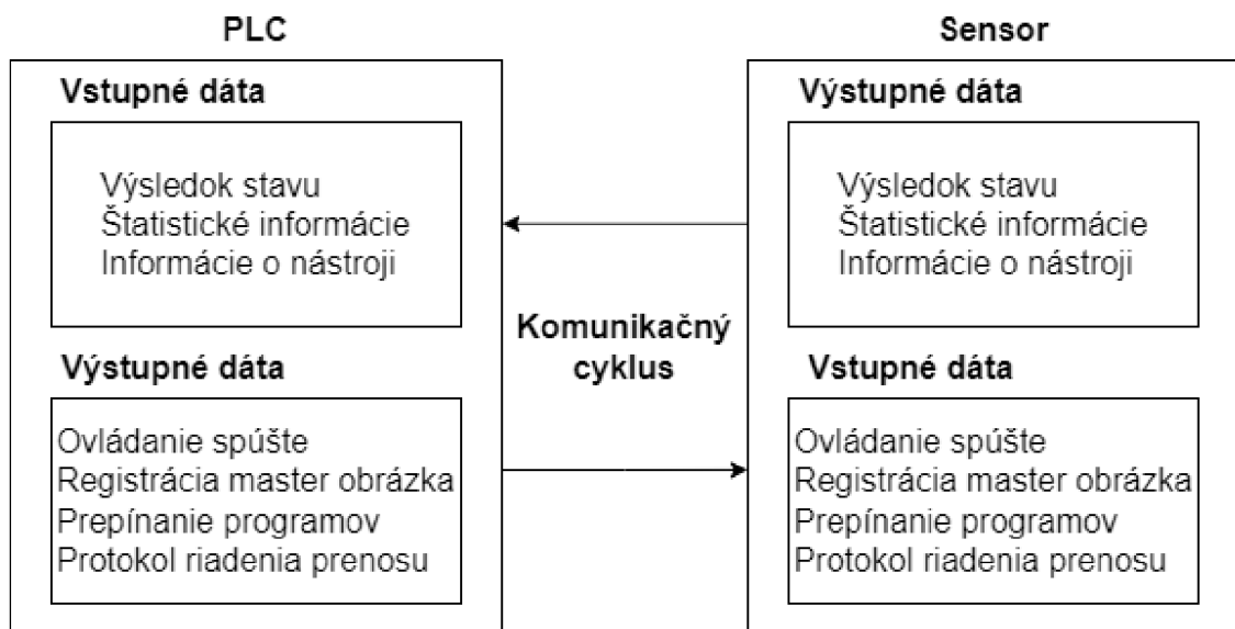
Obr. 3.9: Komunikačný cyklus
