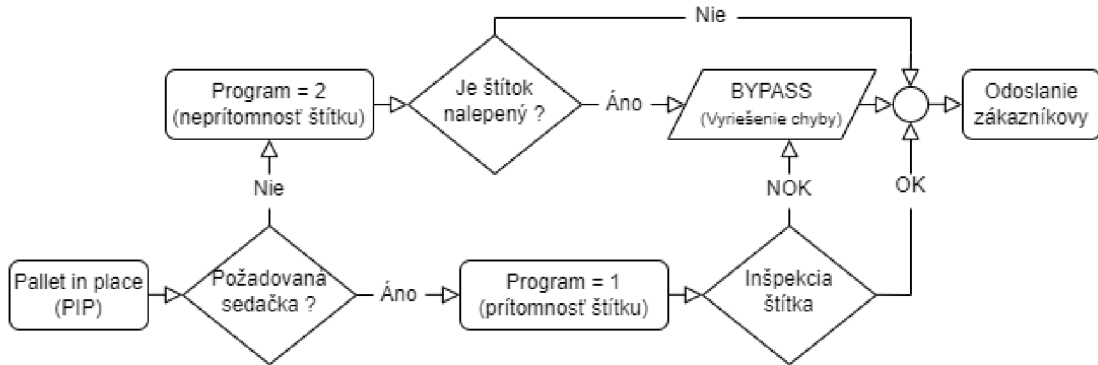
Obr. 4.11: Vývojový diagram programu
