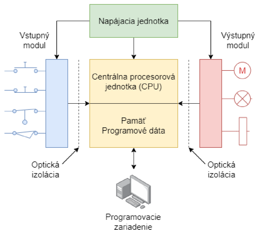
Obr. 1.2: Architektúra PLC [10]
