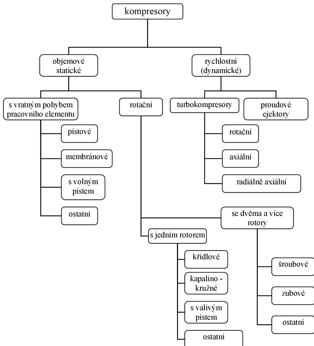
Obr. 1.2 Rozdělení kompresorů podle způsobu stlačování (1)
