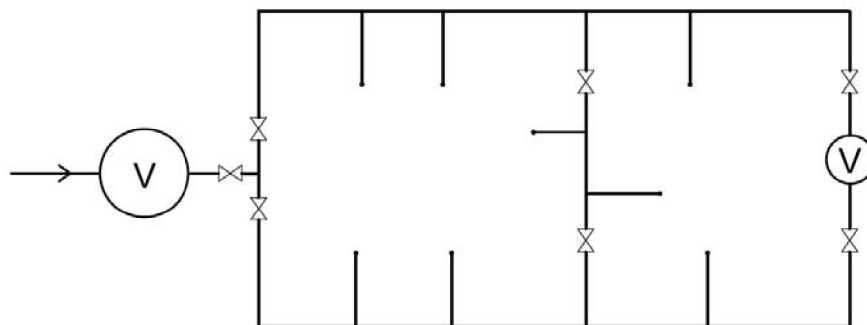
Obr. 2.1 Schéma okružního rozvodu (1)
