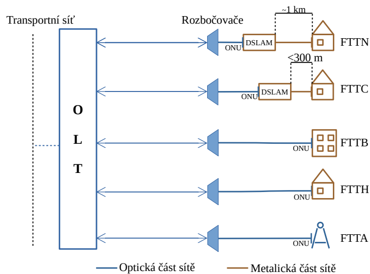
Obr. 9.1: Grafické znázornění FTTx
