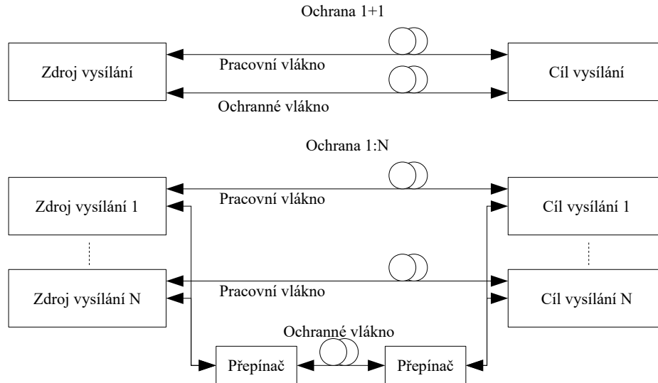
Obr. 2.6: Porovnání ochrany přepínání [5]
