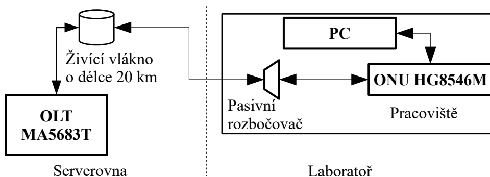
Obr. 6.5: Schéma zapojení laboratorní sítě GPON
