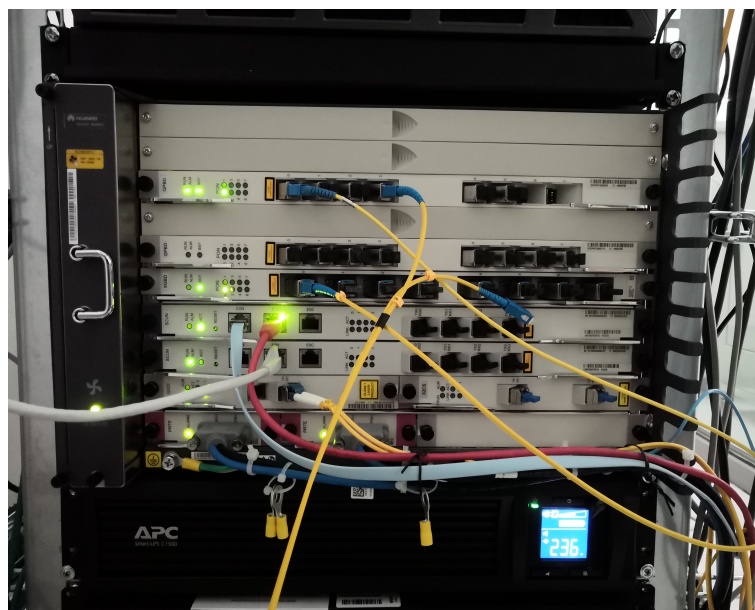
Obr. 9.6: Fotografie OLT platformy MA5683T
