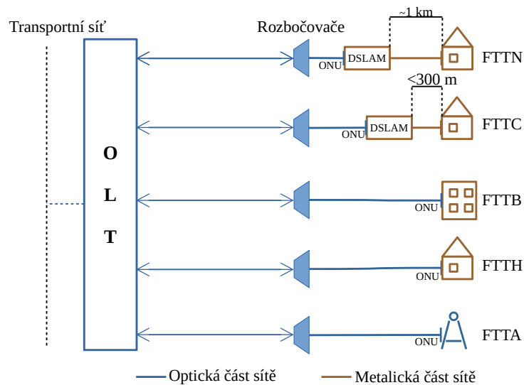
Obr. 7.1: Grafické znázornění FTTx
