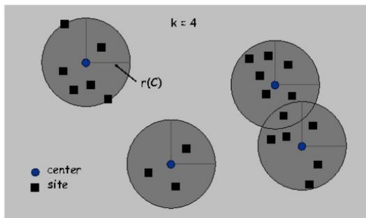
Obrázek 19: k-centers [4]
