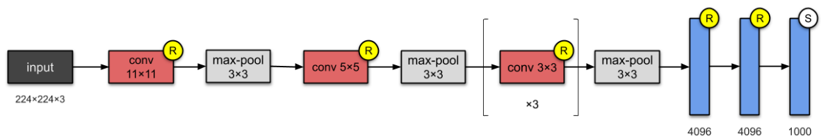
Obrázek 37: AlexNet architektura [13]
