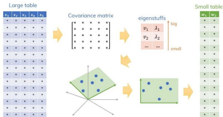
Obrázek 22: PCA algoritmus [3]
