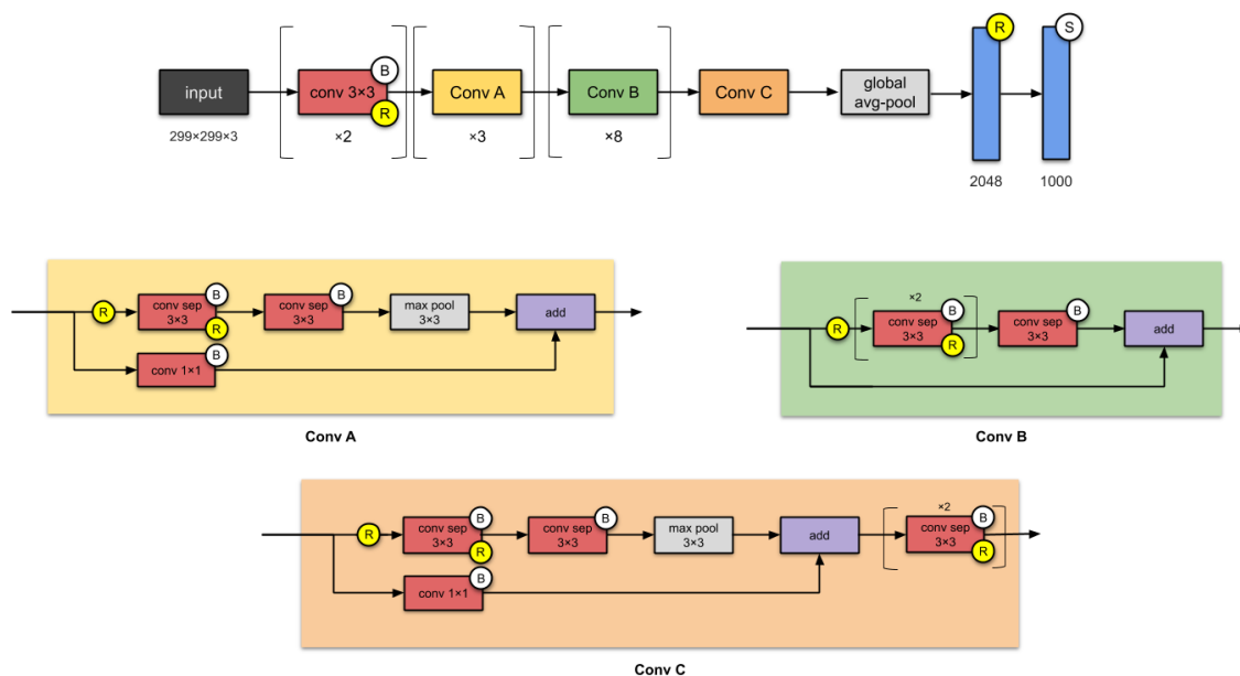
Obrázek 41: Xception architektura [13]
