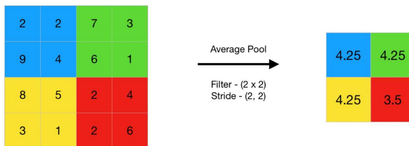
Obrázek 31: average pooling [16]
