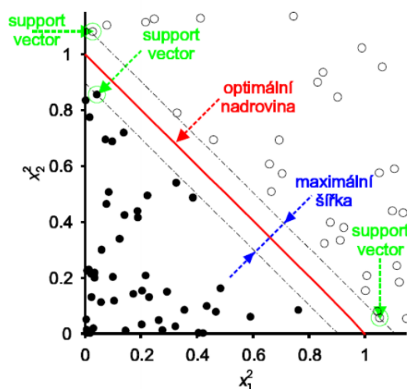
Obrázek 11: ukázka OSVM [10]
