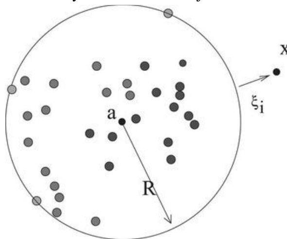
Obrázek 15: SVDD metoda [1]
