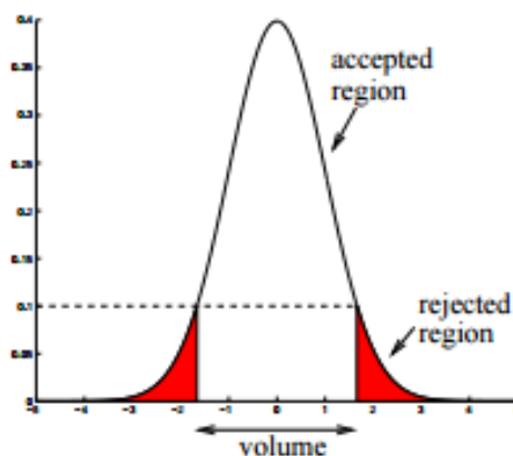
Obrázek 12: Gaussův model [2]
