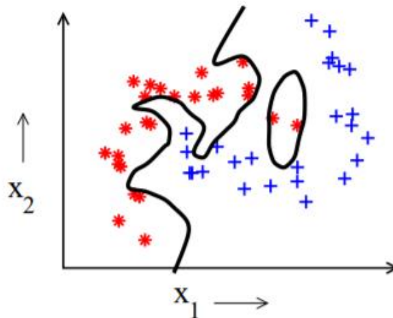
Obrázek 4: Přetrénovaný model [2]
