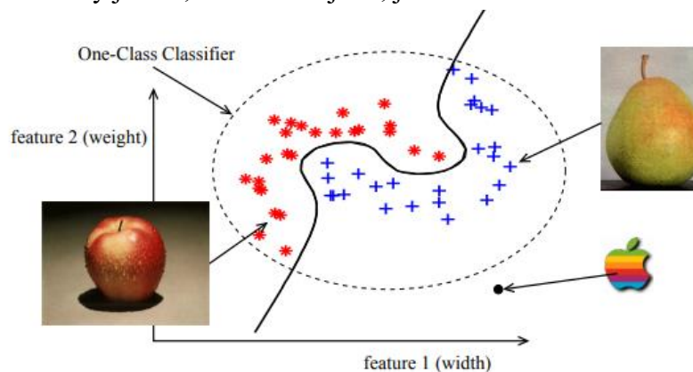
Obrázek 1: Příklad klasifikace [2]
