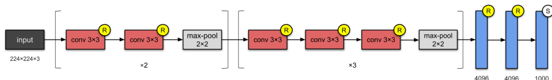
Obrázek 38: VGG-16 architektura [13]
