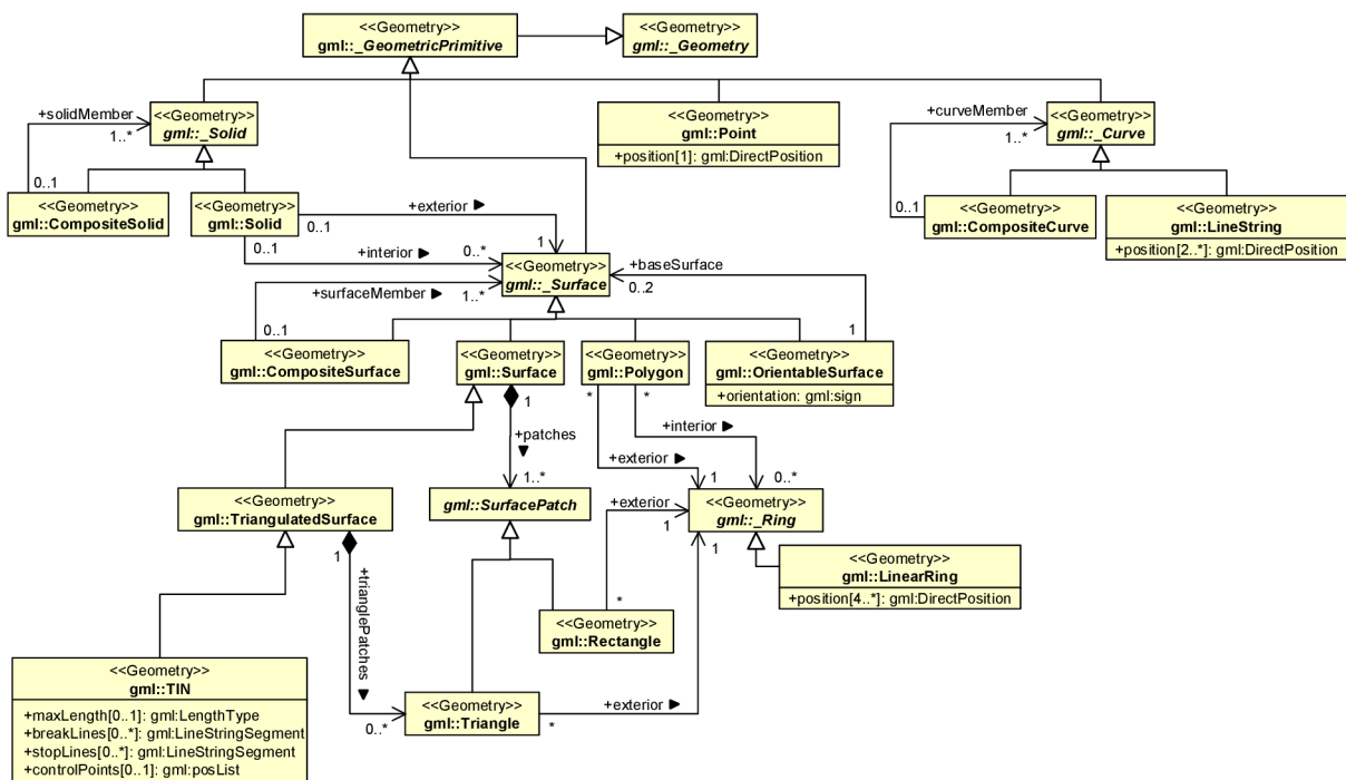
Obr. 5.8 UML diagram CityGML geometrického modelu [28]
