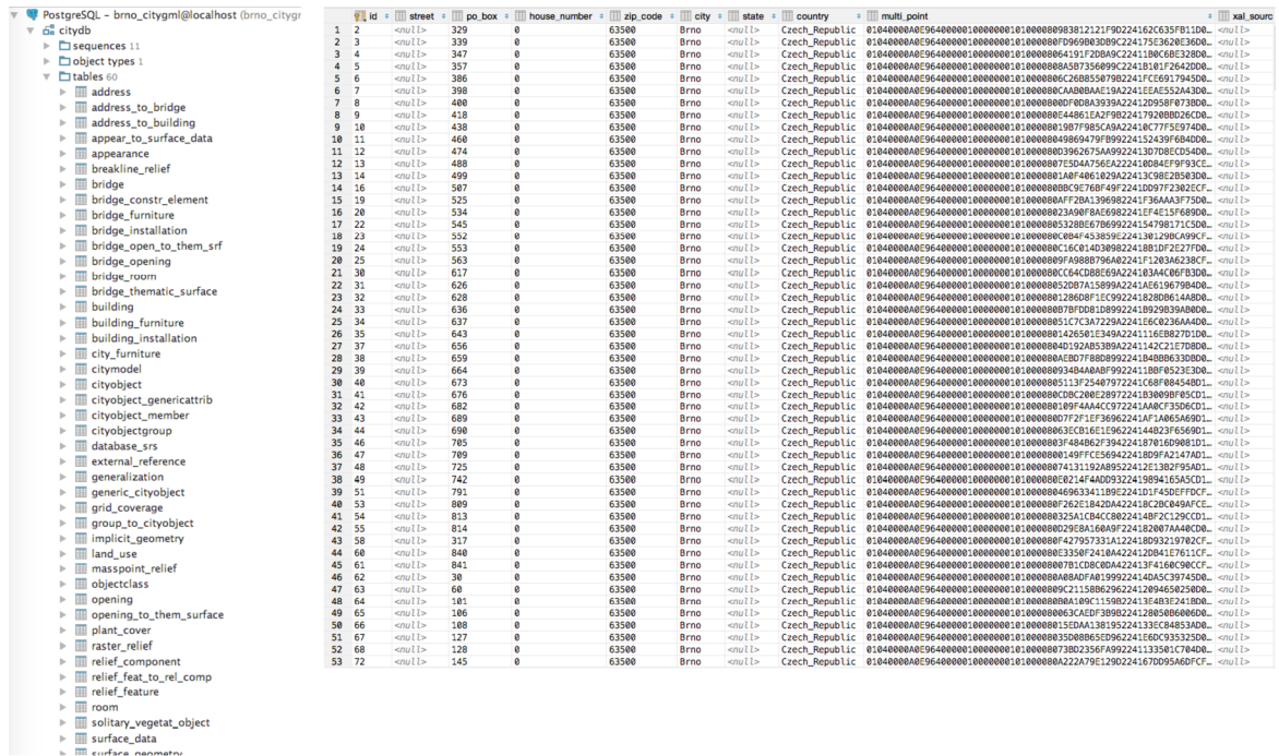
Obr. 6.19 Vľavo – databázová schéma citydb . Vpravo – Tabuľka address , v ktorej sa nachádzajú adresy jednotlivých budov.
