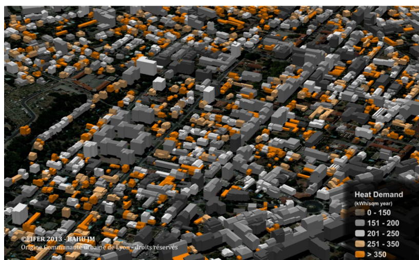
Obr. 4.3 Grafická reprezentácia tepelných strát [23]
