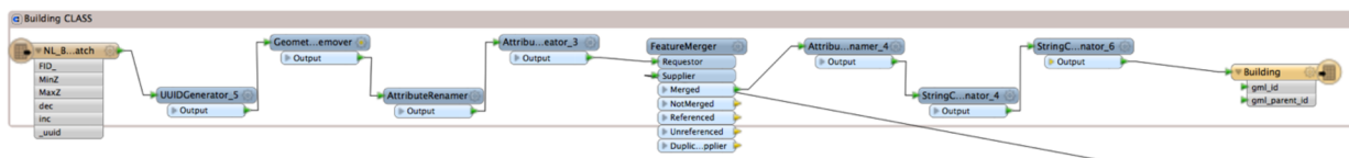
Obr. 6.12 Proces tvorby abstraktnej triedy Building
