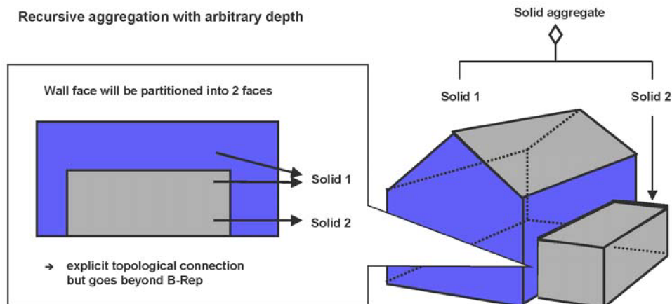
Obr. 5.9 Geometricko-topologický model [28]
