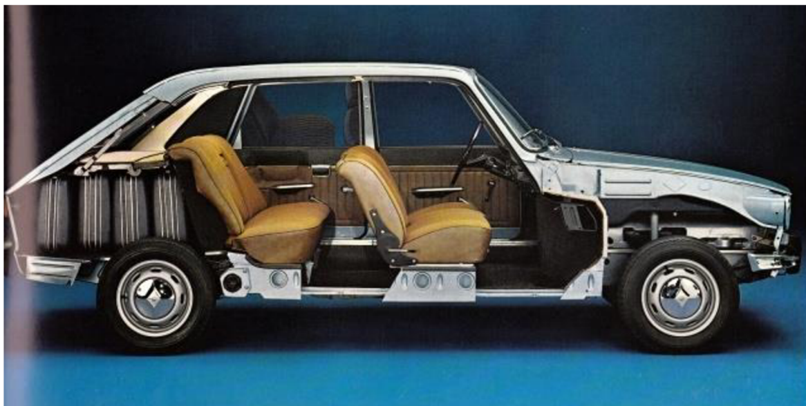
Obrázek 9. Renault 16, [58]
