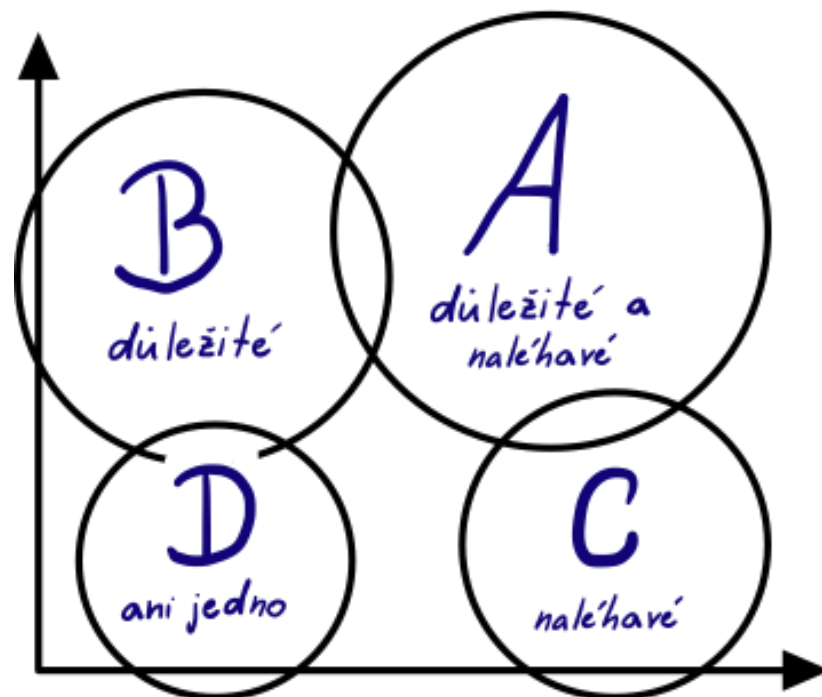
Obrázek 1: Eisenhowerův princip
