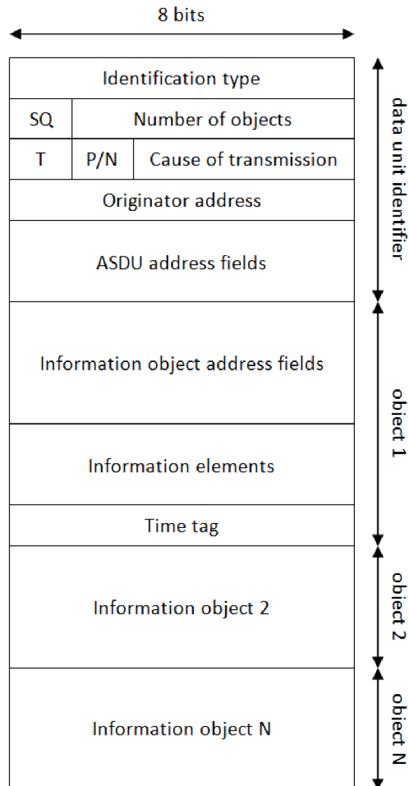
Obr. 1.5: Struktura ASDU.
