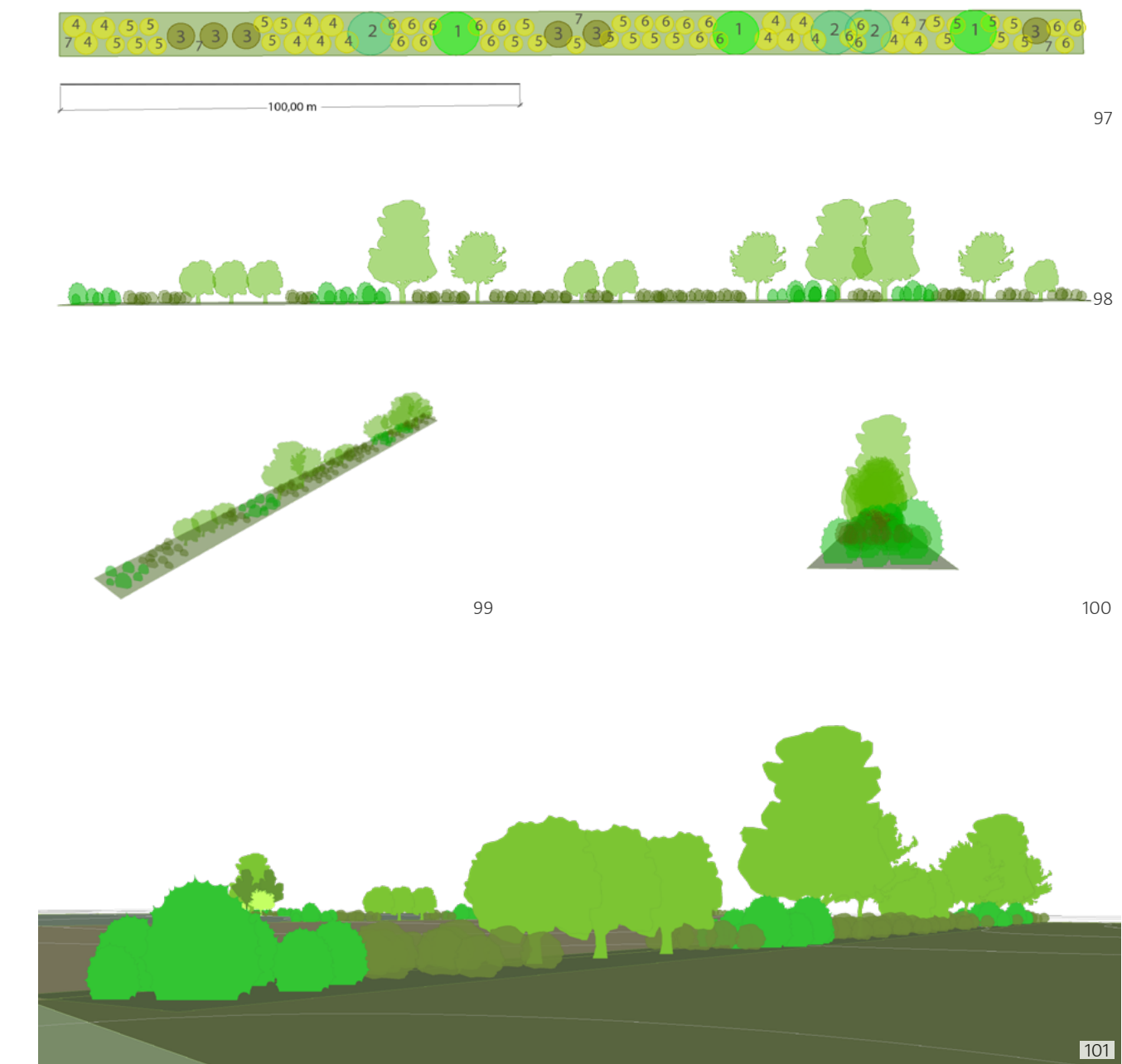
Obrázek 97-101 Liniová zeleň-půdorys, frontální pohled, axonometrie, boční pohled a perspektiva (zdroj viz kapitola 8)
