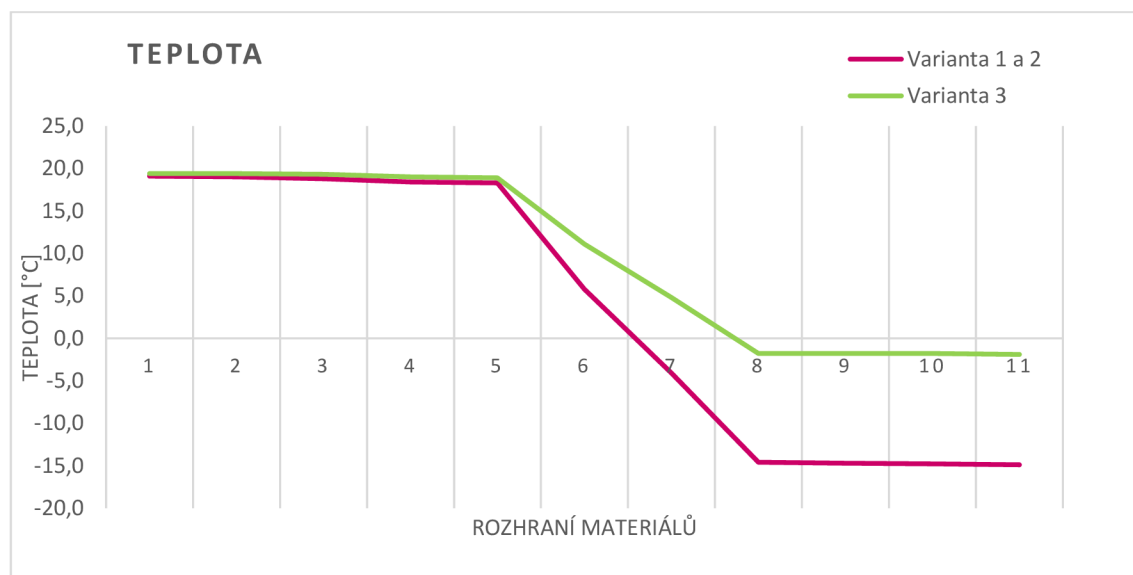
Graf 11 Teplota
