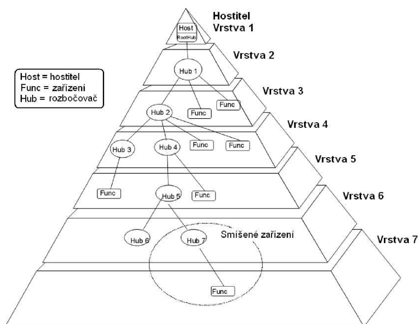
Obr. 2 Stromová struktura sběrnice USB
