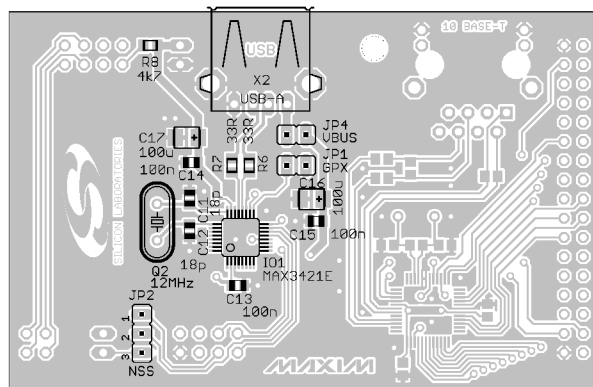
Obr. 28 Osazení součástek na horní straně desky s plošnými spoji modulu USB
