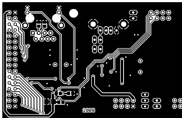
Obr. 27 Spodní strana desky s plošnými spoji modulu USB (1:1)
