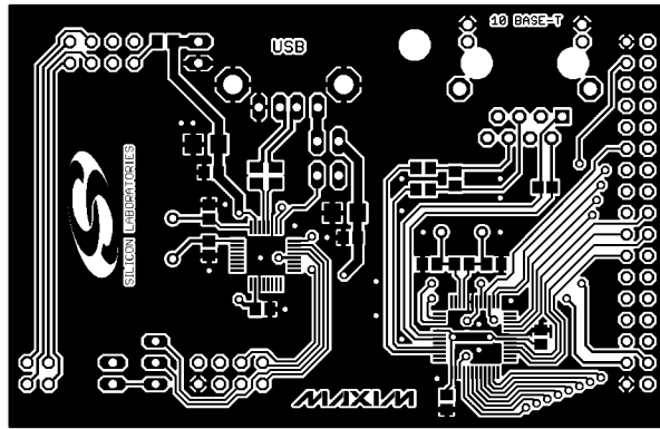
Obr. 26 Horní strana desky s plošnými spoji modulu USB (1:1)
