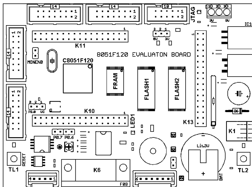
Obr. 24 Rozložení prvků na desce SiLabs C8051F120
