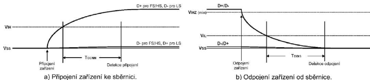
Obr. 4 Časový průběh signálů při připojení a odpojení zařízení
