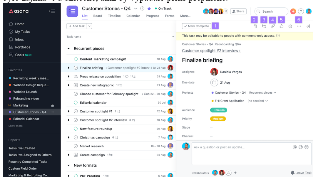
Obrázek 13: Prostředí Asany zdroj: (19)
