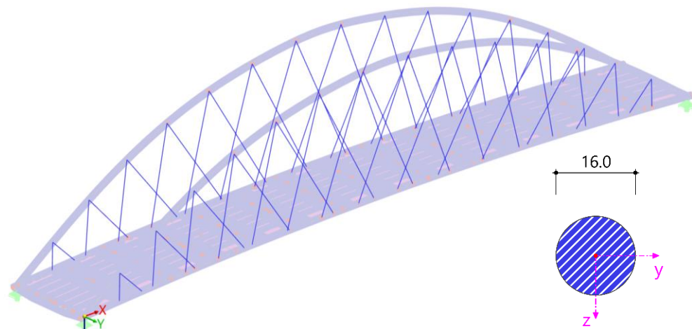
Obr. 10 Táhla
