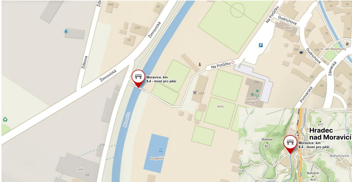
Obr. 1 Umístění lávky
