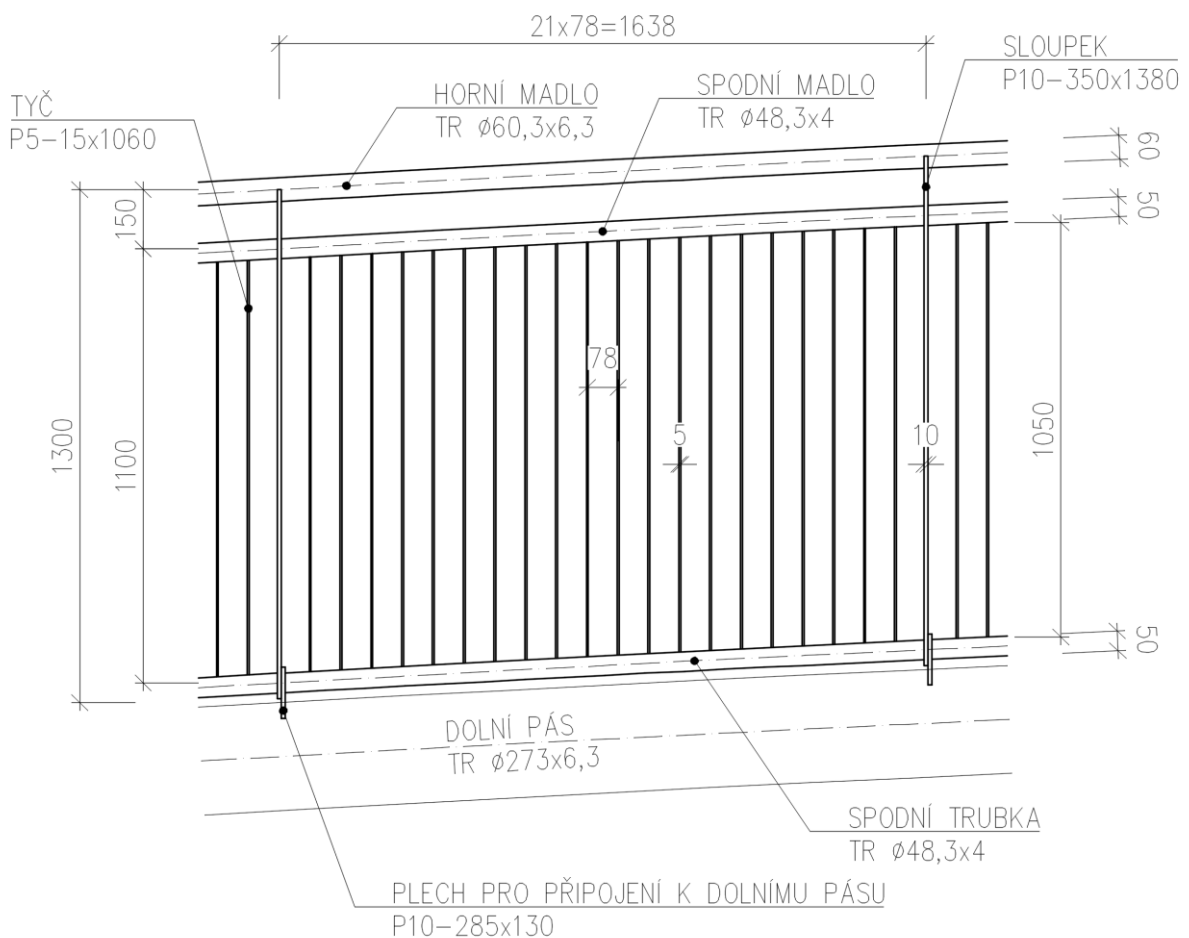
Obr. 16 Zábradlí – pohled na 3. pole
