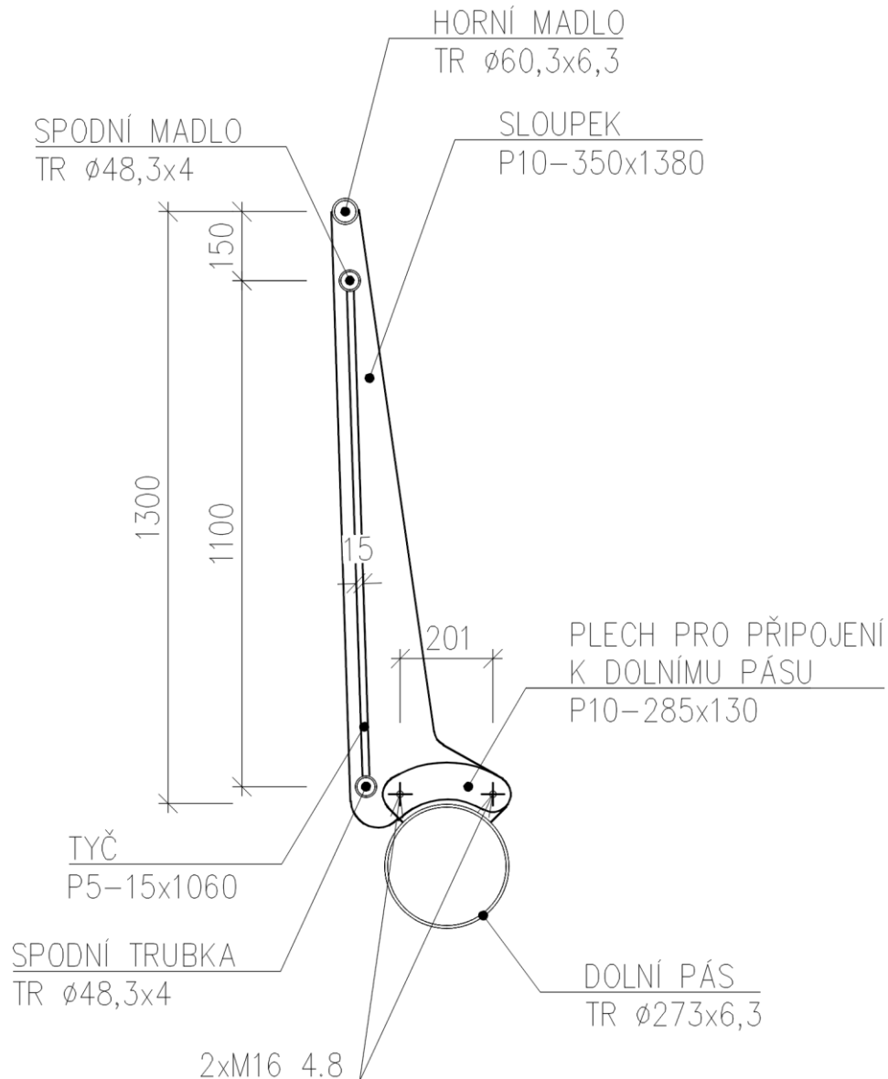
Obr. 17 Zábradlí – příčný řez
