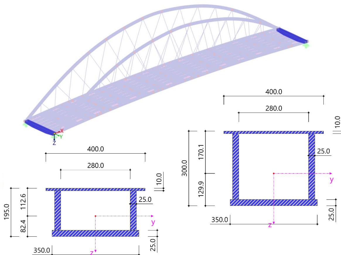
Obr. 14 Krajní příčnický
