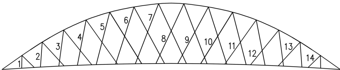
Obr. 9 Konečné uspořádání táhel
