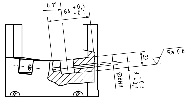
POHLED KOLMO NA DRÁŽKU PRO ULOŽENÍ VÝKYVNÉ UPÍNKY
