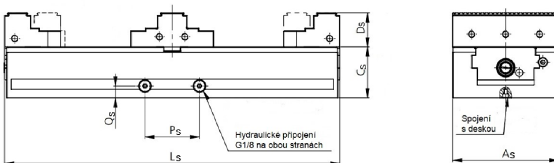
Obrázek 3.18: Schéma svěráku D2 125-H
