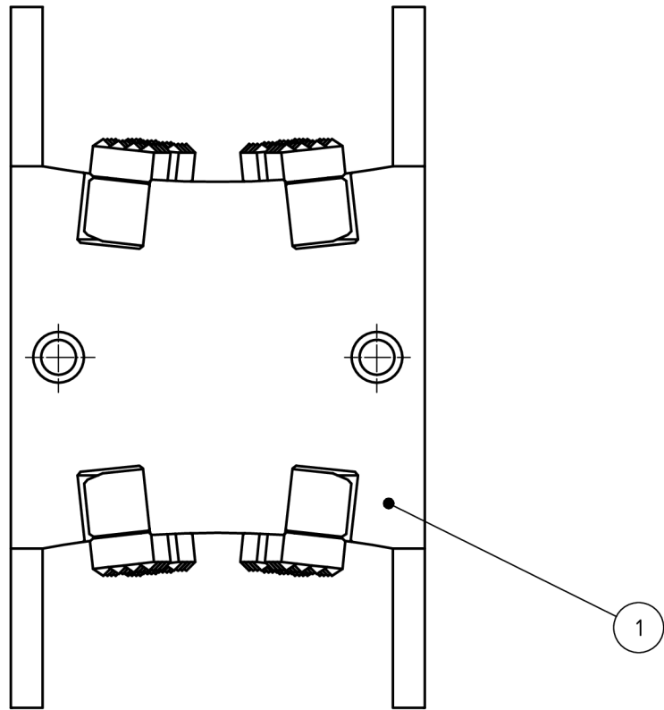
ULOŽENÍ VÝKYVNÉ UPÍNKY V BLOKU ČELISTI (1:1)
