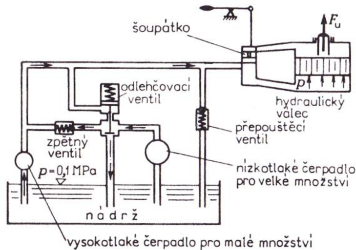
Obrázek 2.8: Hydraulické upínání [8]
