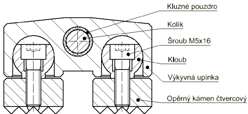
Obrázek 3.8: Uložení opěrných prvků ve výkyvných upínkách. Foto Jan Pokorný
