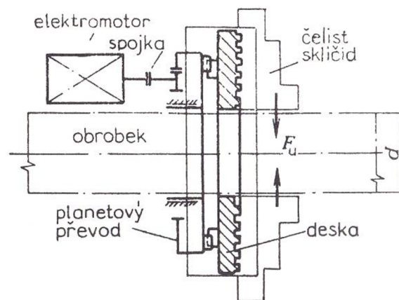
Obrázek 2.6: Elektromechanické sklíčidlo [8]
