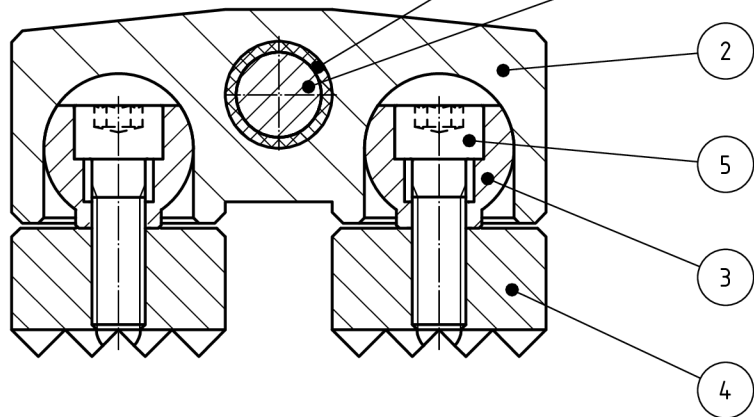
ULOŽENÍ VÝKYVNÉ UPÍNKY V BLOKU ČELISTI (1:1)
