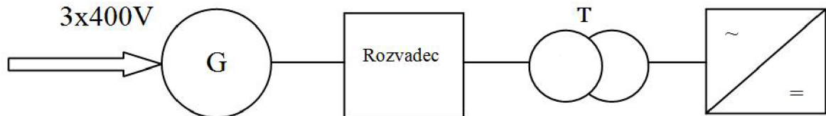
Obr. 3-5 blokové schéma napájení cívek Tokamaku přes generátor, rozvaděč, transformátor a měnič
