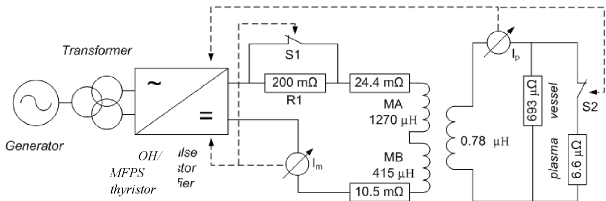
Obr. 3-13 Schéma obvodu OH start [8]
