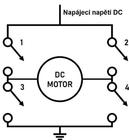
Obrázek 6.9 - Schéma H-můstku [23]
