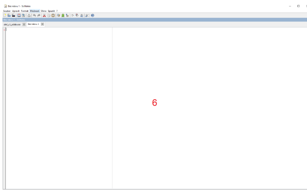
Obrázek 5.2 - Editor SciNotes
