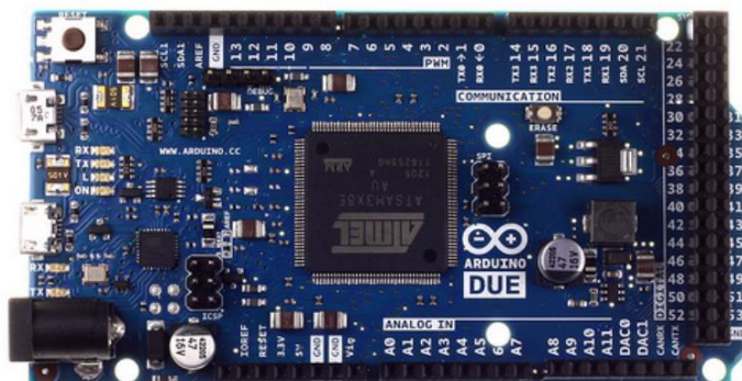
Obrázek 4.9 - Arduino Due [4]
