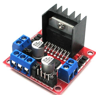
Obrázek 6.8 - H-můstek L298N [22]
