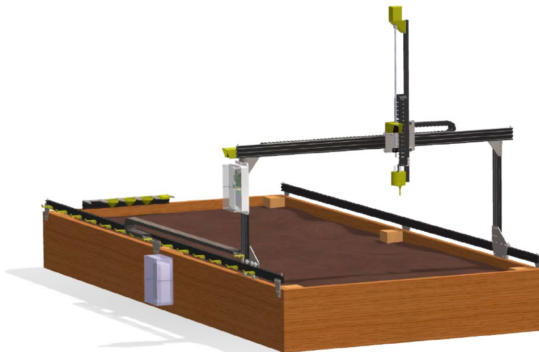
Obrázek 23 Systém Farmbot [15]
