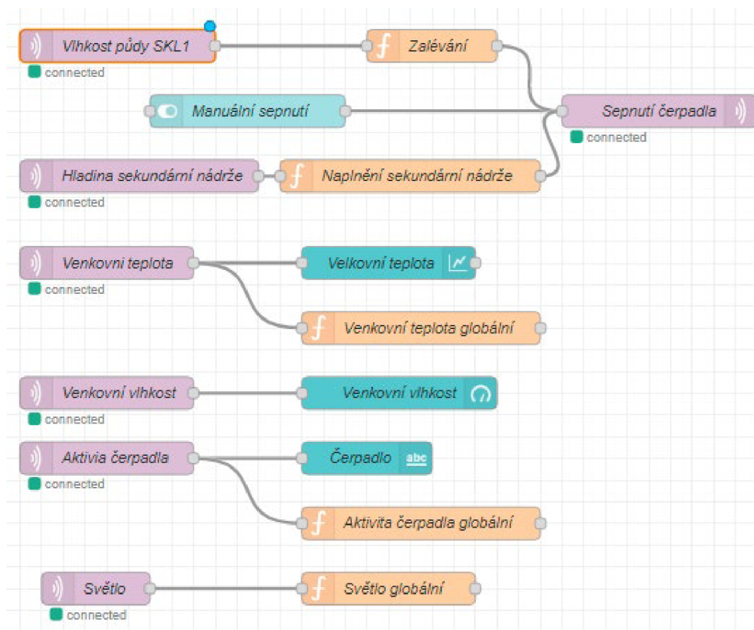
Obrázek 27 Node Red flowes pro Čerpadlo. Zdroj: Vlastní
