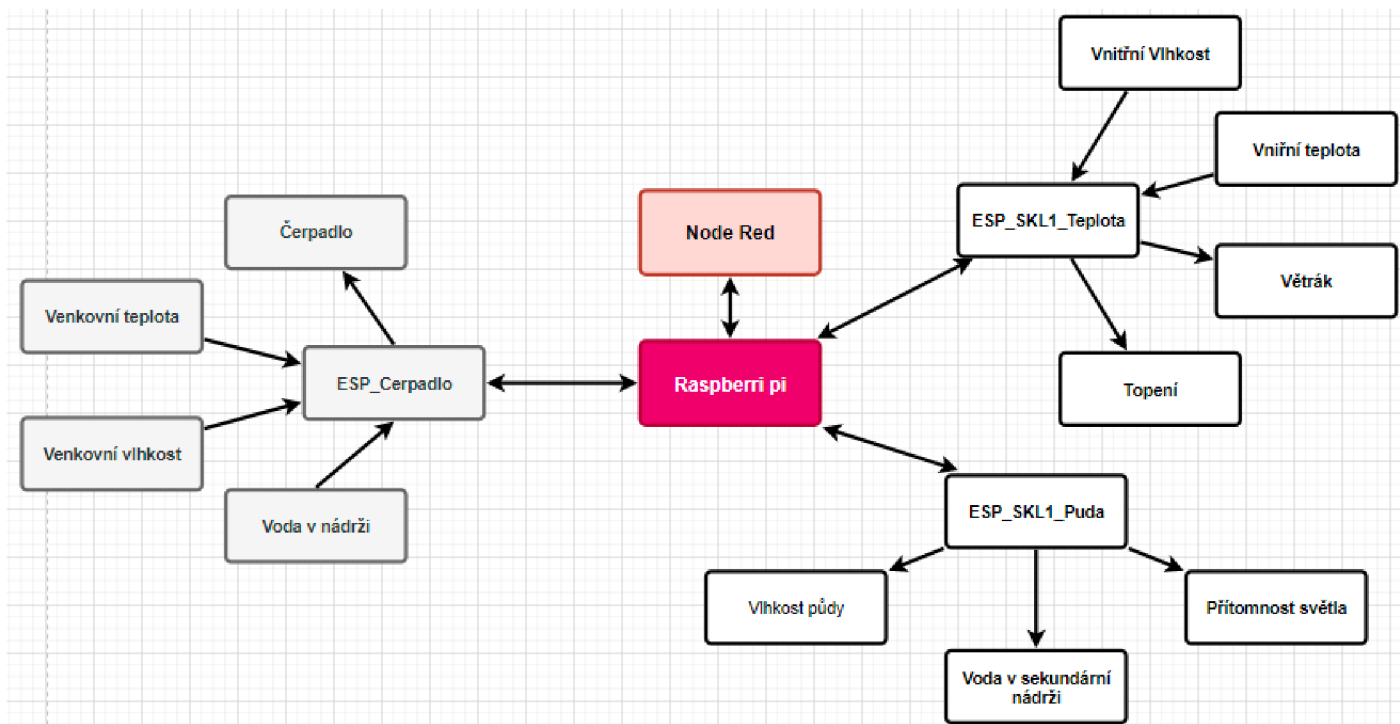
Obrázek 24 Schéma navrženého systému Zdroj: Vlastní
