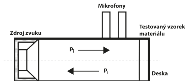
Obr. 5: Schéma impedanční trubice, vlastní zpracování [6, s. 78]
