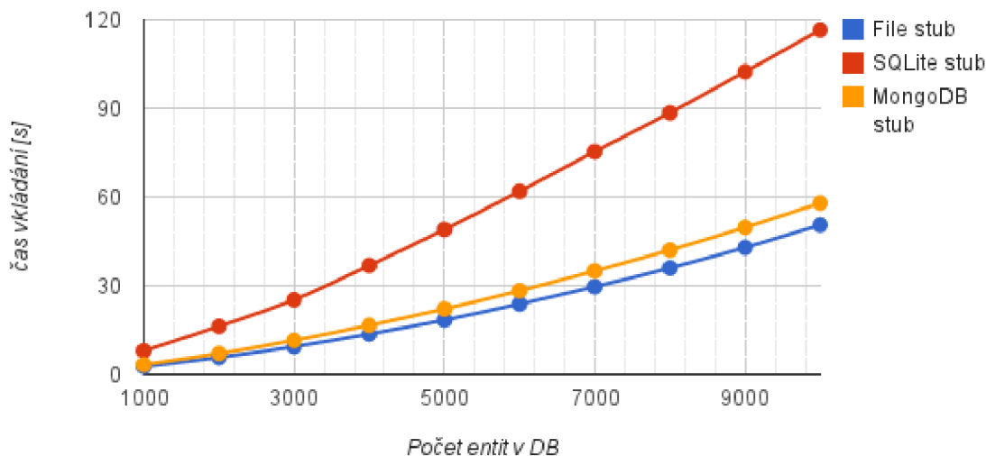
Obrázek 6.1: Srovnání zápisové rychlosti Datastore MongoDB Stubu s existujícími stuby.
