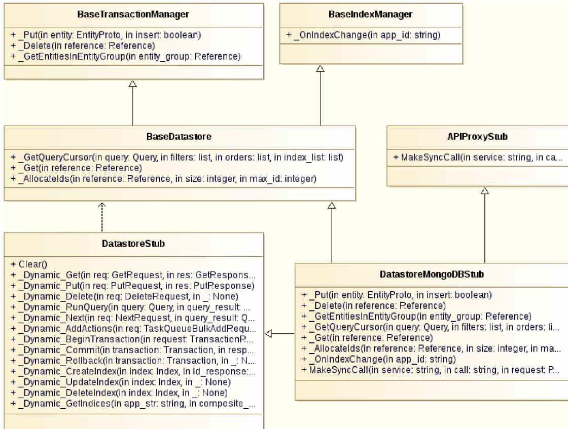
Obrázek 5.1: UML diagram tříd 2 znázorňující stavbu Datastore MongoDB Stubu.
